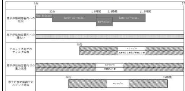
第2-5-3図 放出放射能評価のクロノロジ
