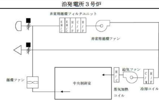
第3回 中央制御室非常用循環系統 概略系統構成
