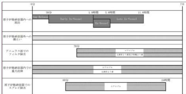
第3図 放出放射能評価のクロノロジ
