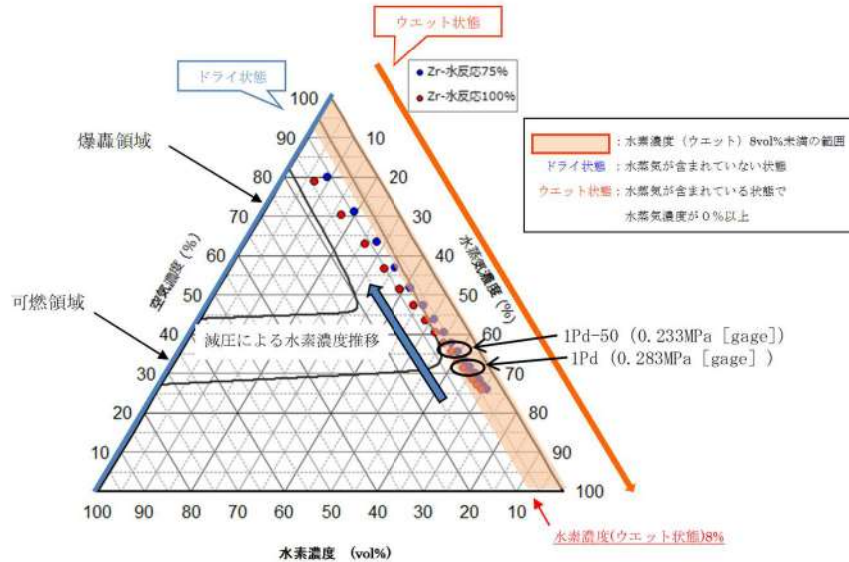
図2 空気、水素、水蒸気の三元図
