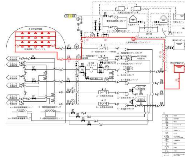
図 49-4-2 代替格納容器スプレィ
