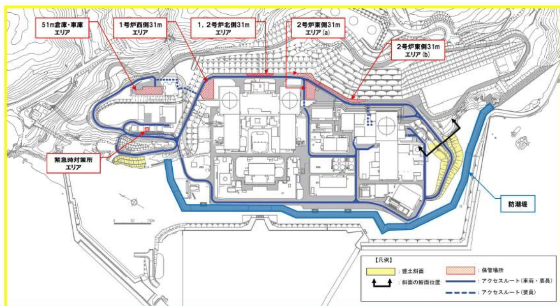
第 4-1 図 盛土斜面平面位置図
