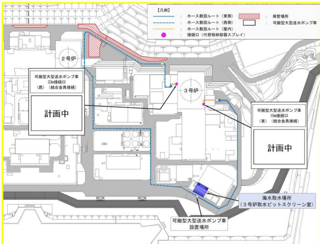
第3図 建屋接続場所(4/8)
