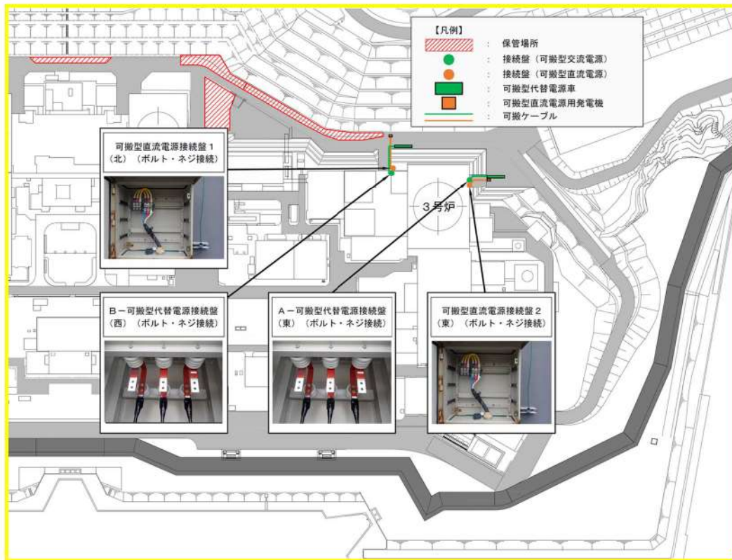
第3図 建屋接続場所(3/8)
