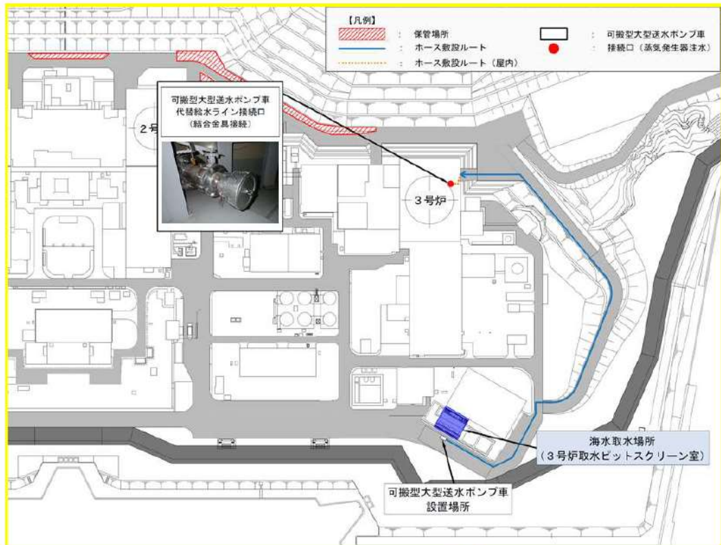
第3図 建屋接続場所(6/8)
