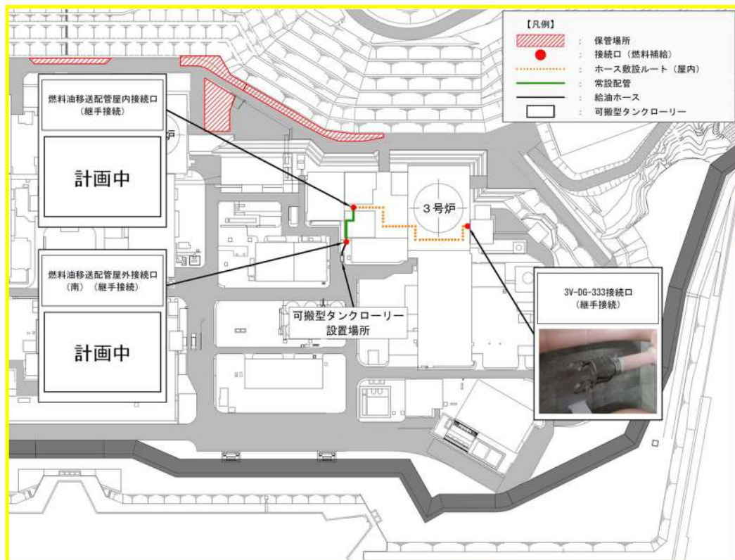
第3図 建屋接続場所(8/8)
