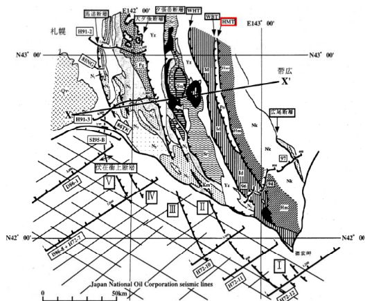
図1 日高衝突帯ならびに前縁褶曲・衝上断層帯の地質概略と主な反射法地震探査測線図。X-X'は図2の断面位置を示す。伊藤ら(1999)を改変。 【地質】主として、地質調査所(1982, 1996)による。Nk: 中の川層群, Hm: 日高変成岩類(主帯), Po: ポロシリ・オフィオライト(西部), Id: イドシナップ帯, Yz: 櫻島層群, Sr: 空知層群, Km: 神威古羅変成岩類, Sn: 沙流川層一セウ層, Pg: 古第三系, N1~N3: 地質調査所(1982)に同じ, Qv: 第四紀火山岩類, [HMT: 日高主衝上断層], WBT: 西縁衝上断層, WHT: 日高西部断層群 【測線】94・96・97: 日高深部構造反射法探査, 85NG・86TK: 浅野ら(1990), Y97: 佐藤ら(1998), その他の測線は石油公団(1973, 1987, 1993, 1996)。
