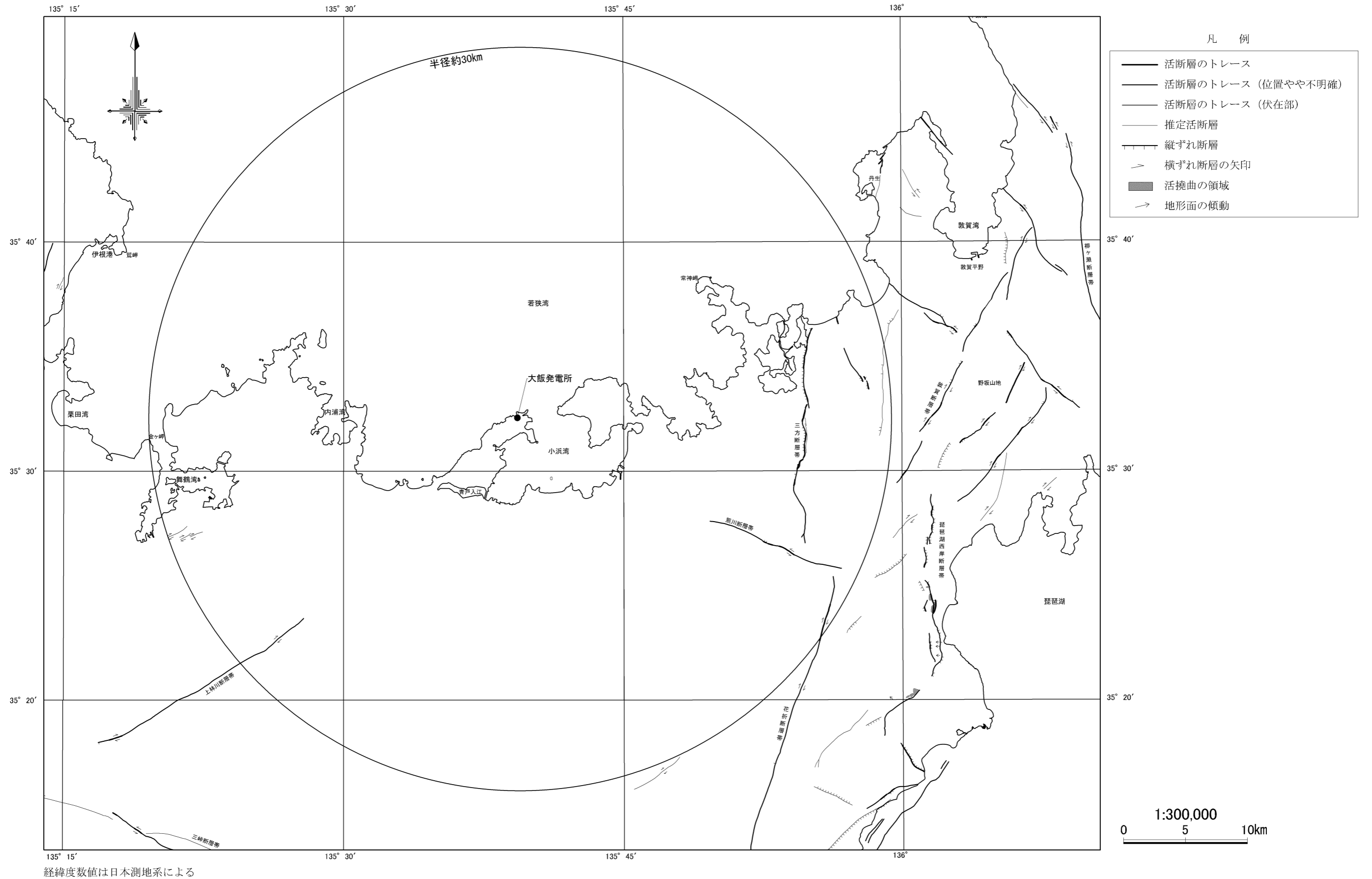
第1.2.3.1.5図 敷地周辺陸域の活断層分布図 「活断層詳細デジタルマップ [新編]」
