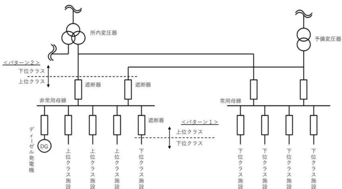
第5.2-1図 受電系統概念図
