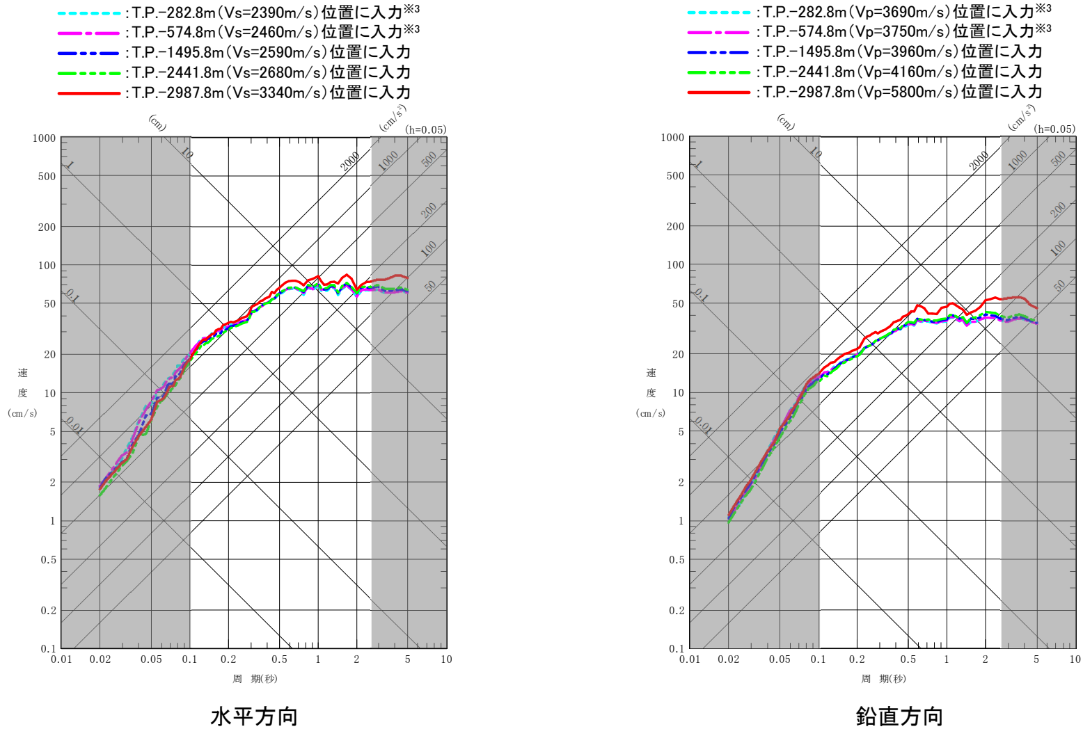
図1 各入力位置による解放基盤表面における地震動(応答スペクトル) ※4
