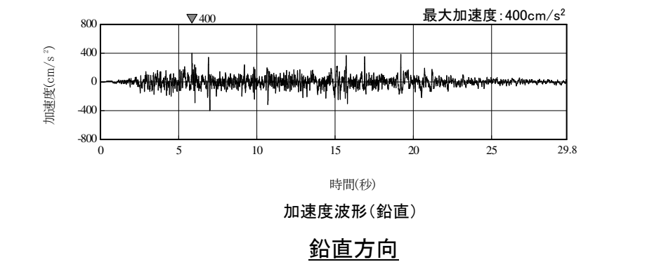
地震基盤相当面における標準応答スペクトルに適合する模擬地震波
