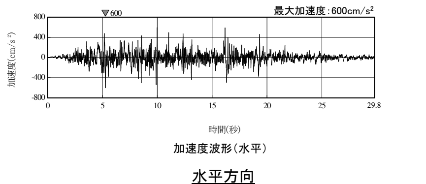
地震基盤相当面における標準応答スペクトルに適合する模擬地震波
