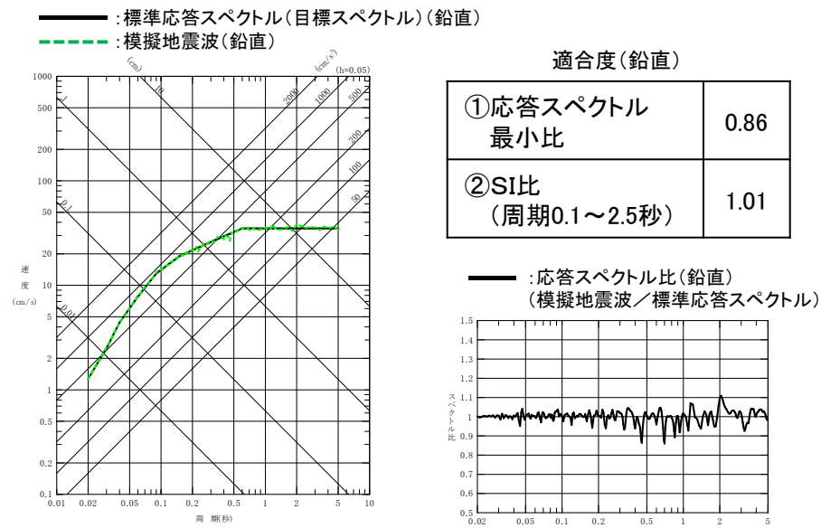
標準応答スペクトルと 模擬地震波の応答スペクトル(鉛直)
