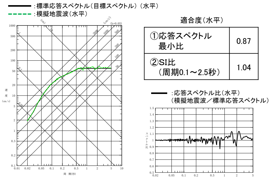
標準応答スペクトルと 模擬地震波の応答スペクトル(水平)
