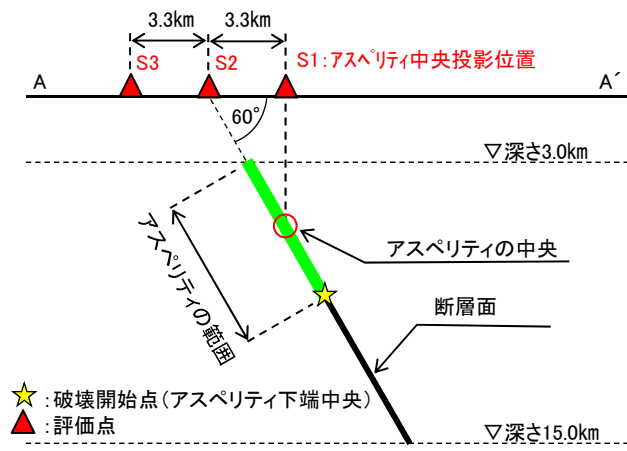
評価点の配置図(A-A'断面)
