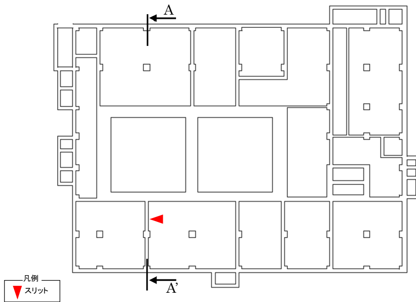
図1 2階床伏図
