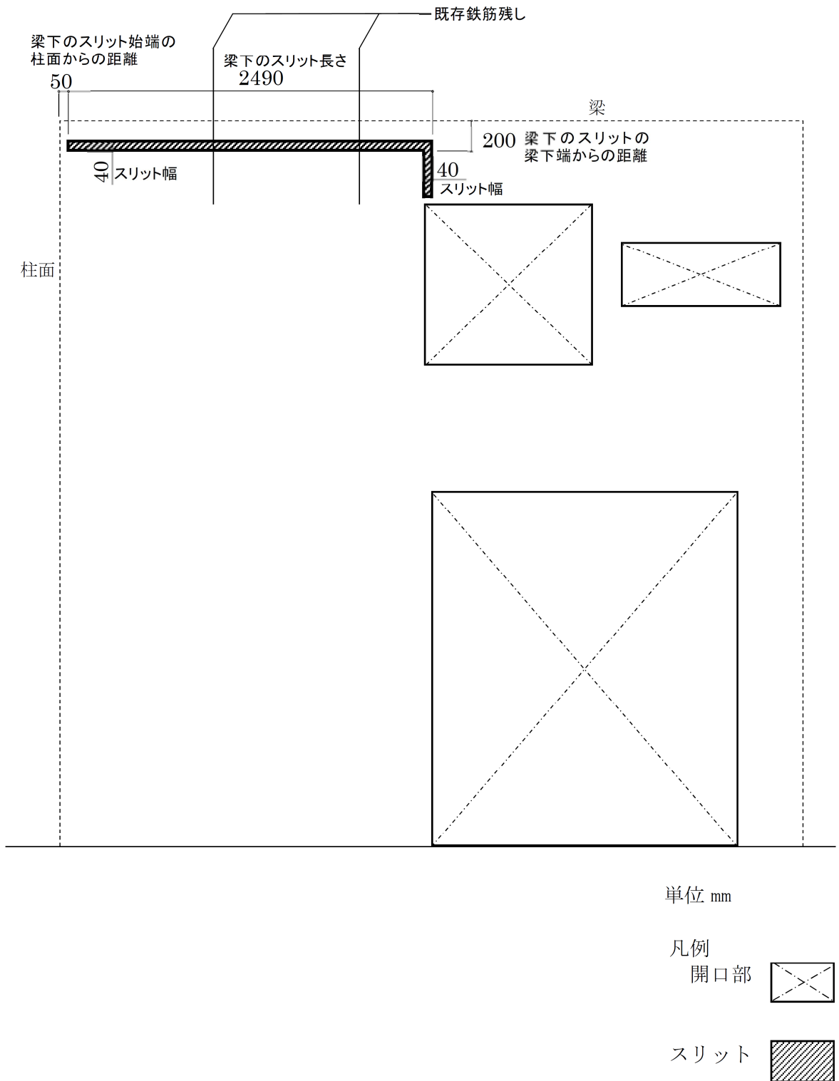
図3 耐震スリット構造 (B 詳細図)
