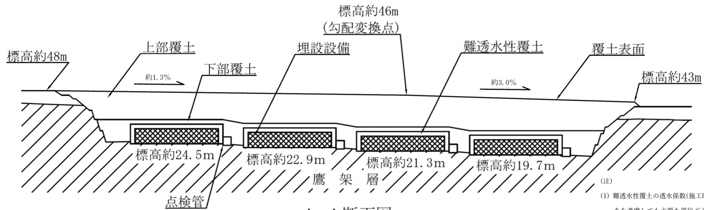
A-A断面図
