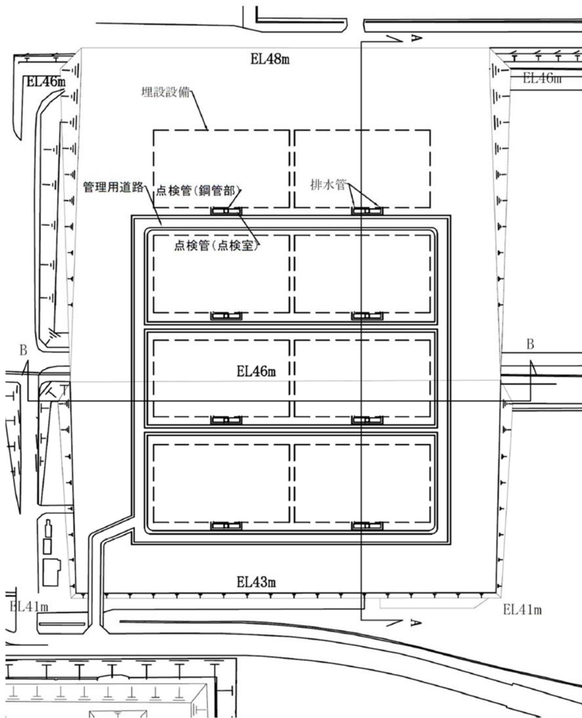
図 1-イ(イ)-1 廃棄物埋設地の設計図(1)
