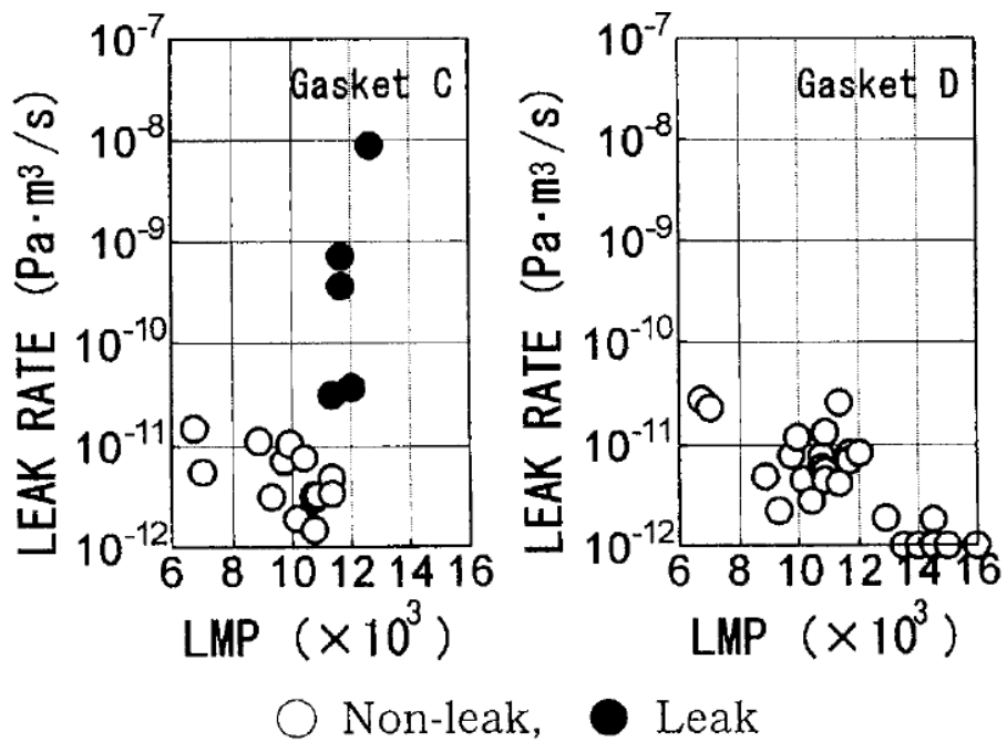
第 1-19 図 漏えい率と LMP の関係 (定数 C=20) (16)
