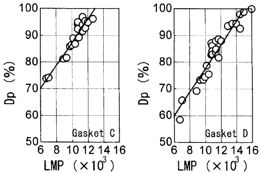
第 1-17 図 塑性変形率 D_p と LMP の関係 (16)
