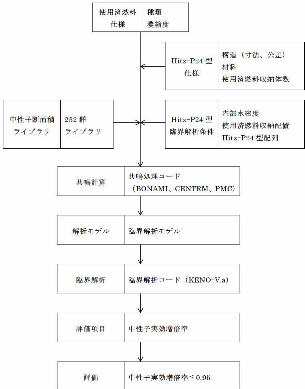
第 1-5 図 臨界解析フロー図
