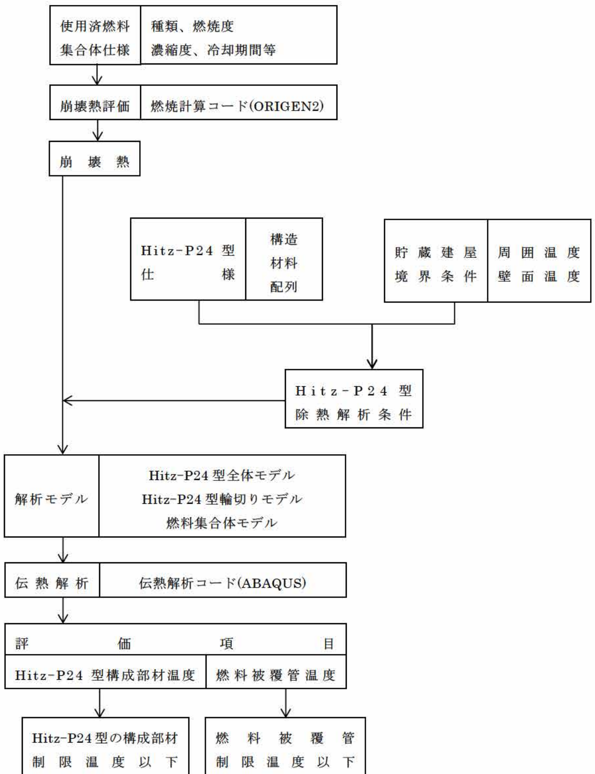
第 1-9 図 除熱解析フロー図
