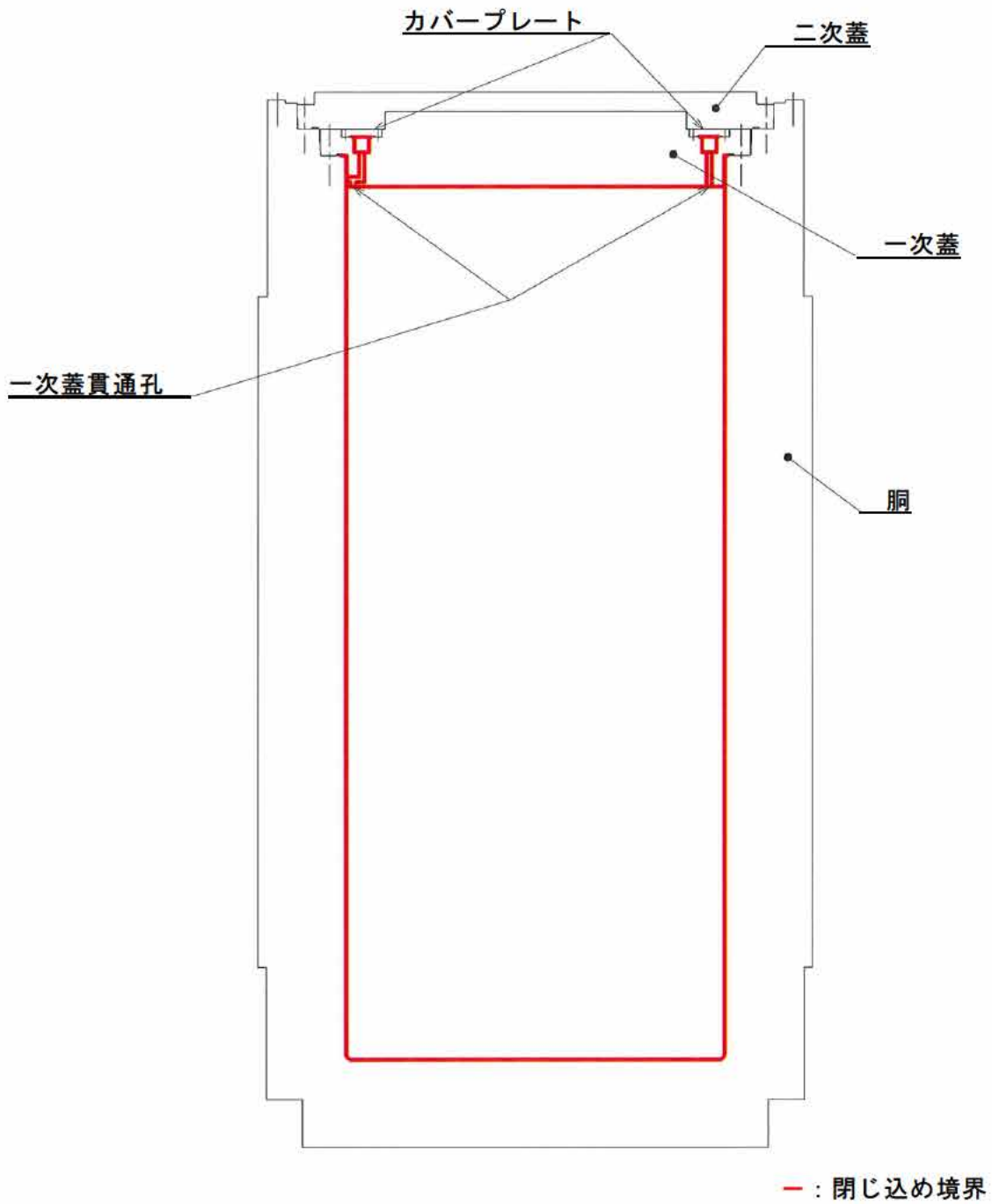
第 1-11 図 Hitz-P24 型の閉じ込め構造
