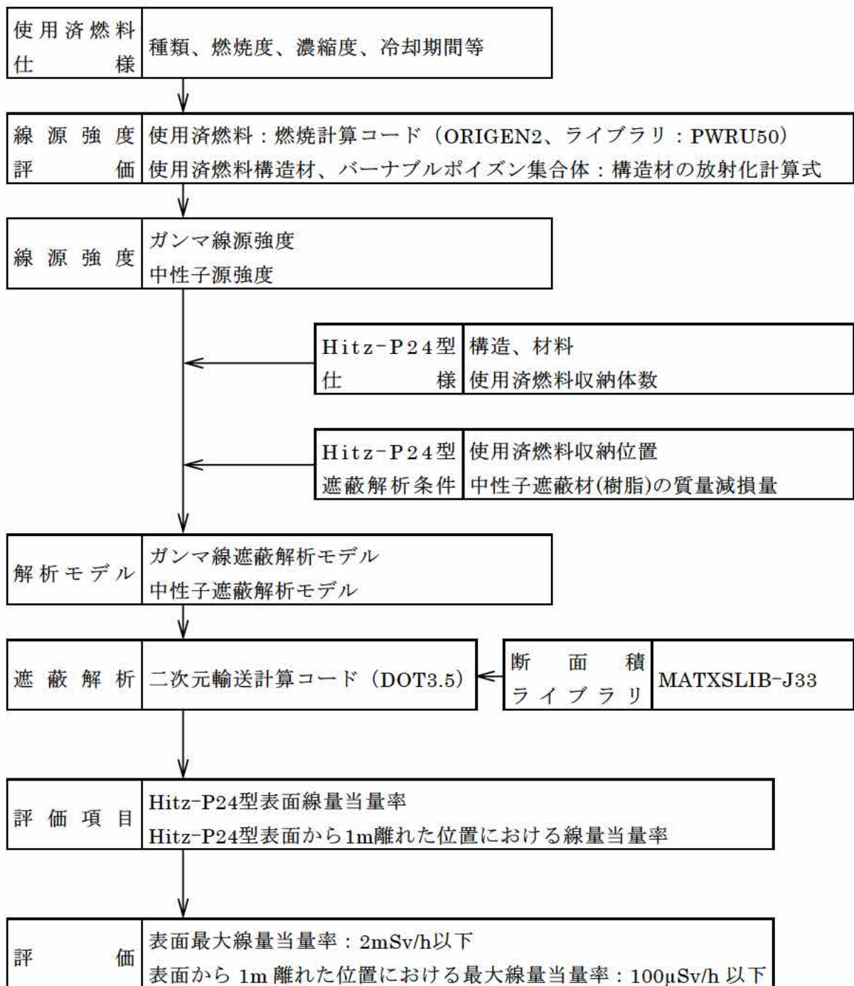
第 1-6 図 遮蔽解析フロー図
