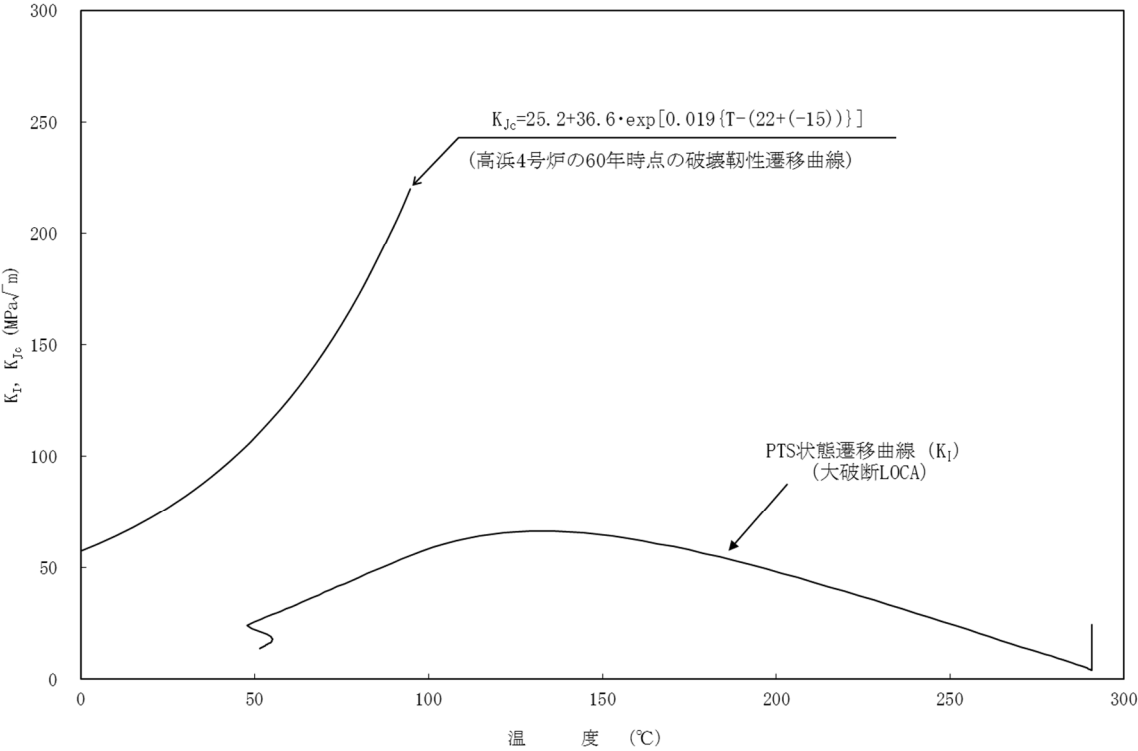
図 参考 1-1 JEAC4206-2016 を用いた PTS 評価結果
