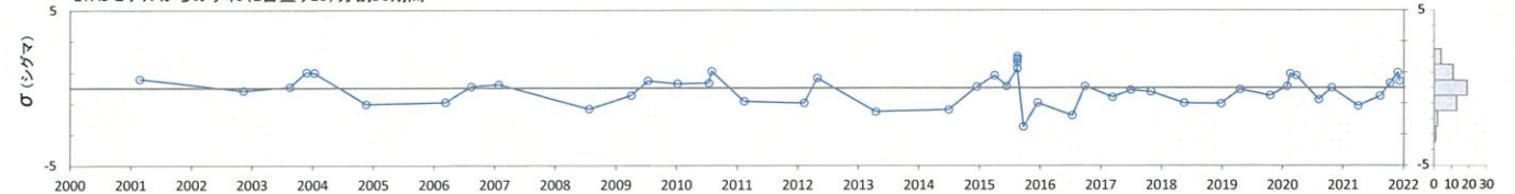
ETASモデルからのずれ(1日盛り1 \sigma )分割50期間
