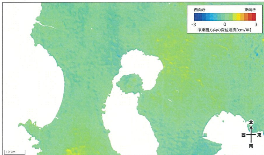
変位速度(cm/年) (準東西方向)
