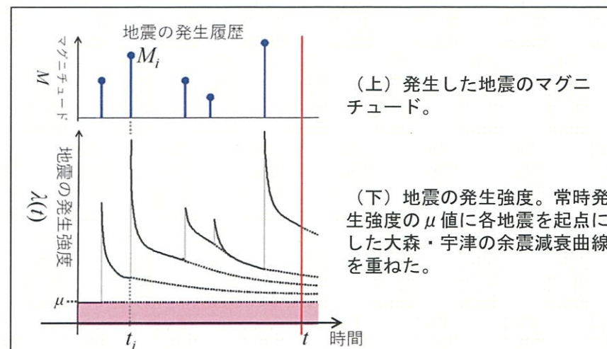
ETASモデルの模式図 (日本地震学会広報誌「なみふる」第117号)
