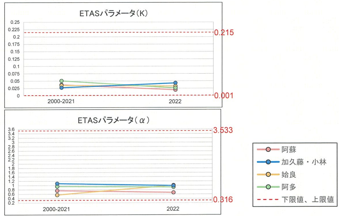
文献(宇津, 1999; 石垣, 2009)で求められているETASモデルのパラメータ範囲
