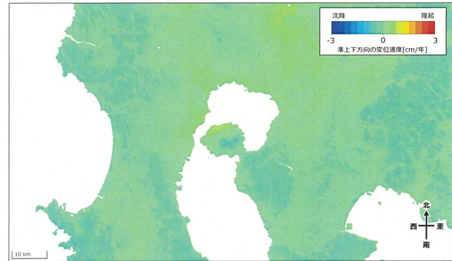
変位速度(cm/年) (準上下方向)
