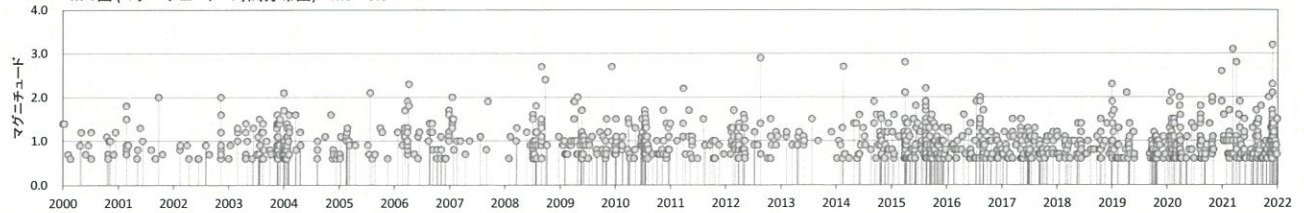
ETASモデルからのずれ(1日盛り1 \sigma )分割50期間
