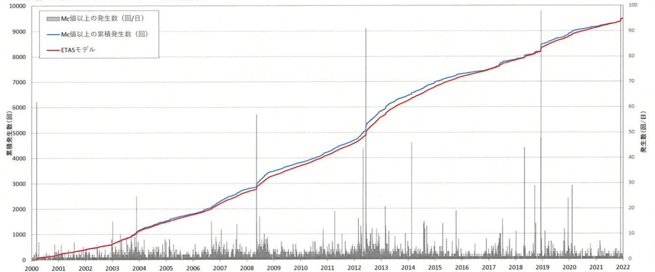
M-T図 (マグニチュード・時間分布図) M_c=0.3
