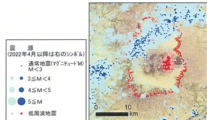
震源分布(深さ50km以浅)
