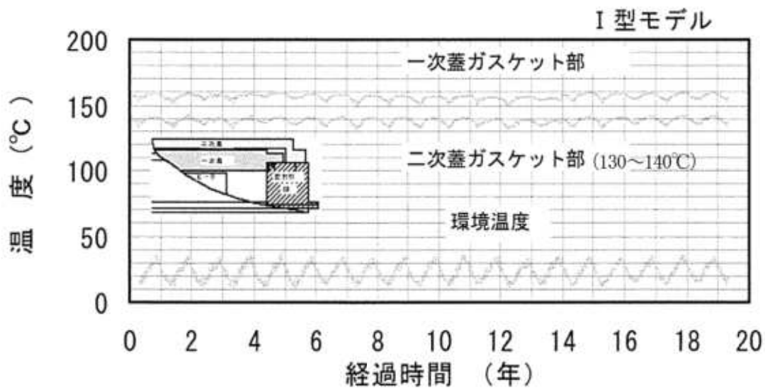
第7図 金属ガスケット（二次蓋）の長期密封性能試験結果（眼鏡型） ②
