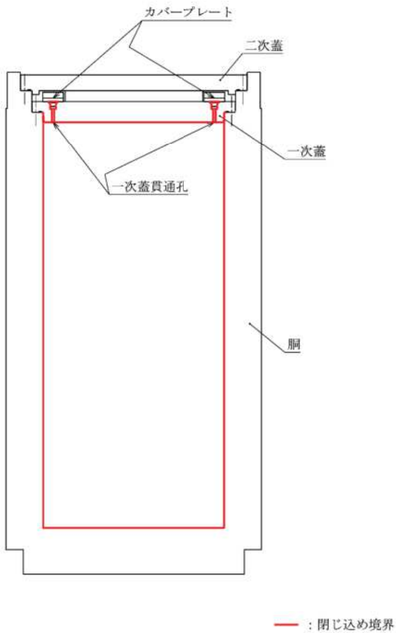
第1図(2/2) MSF-28P型の閉じ込め構造 (基礎等に固定する設置方法)
