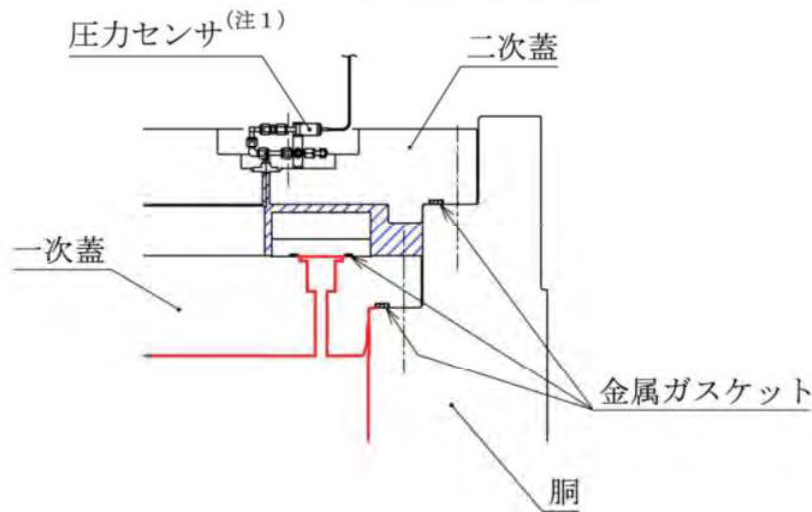
閉じ込め機能の監視構造
