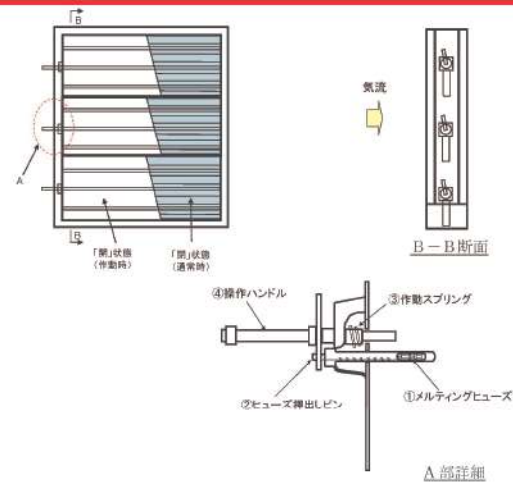
図1-5 ダクト開放機構概略図
