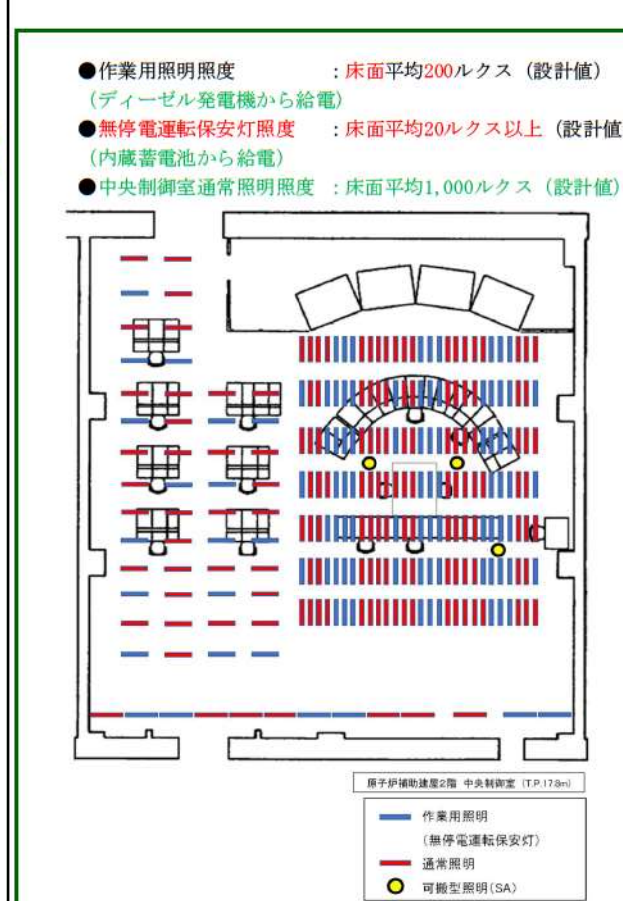
図2.5-2 中央制御室照明設備の概要図
