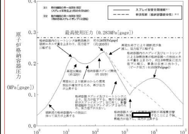
図2.1.3.10 スプレィ立上り配管の全周破断を想定した場合の格納容器内圧力 (スプレィ流量として安全解析で考慮している値の36%の場合)
