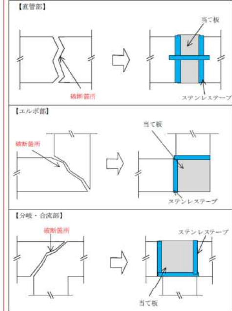
第2.1.2.3図 当て板による修復イメージ
