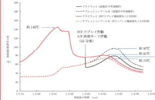
図2.1.3-2 原子炉格納容器健全性解析結果 (プレッションプール冷却モード作動)
