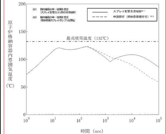
図2.1.3.11 スプレィ立上り配管の全周破断を想定した場合の格納容器内雰囲気温度 (スプレィ流量として安全解析で考慮している値の36%の場合)
