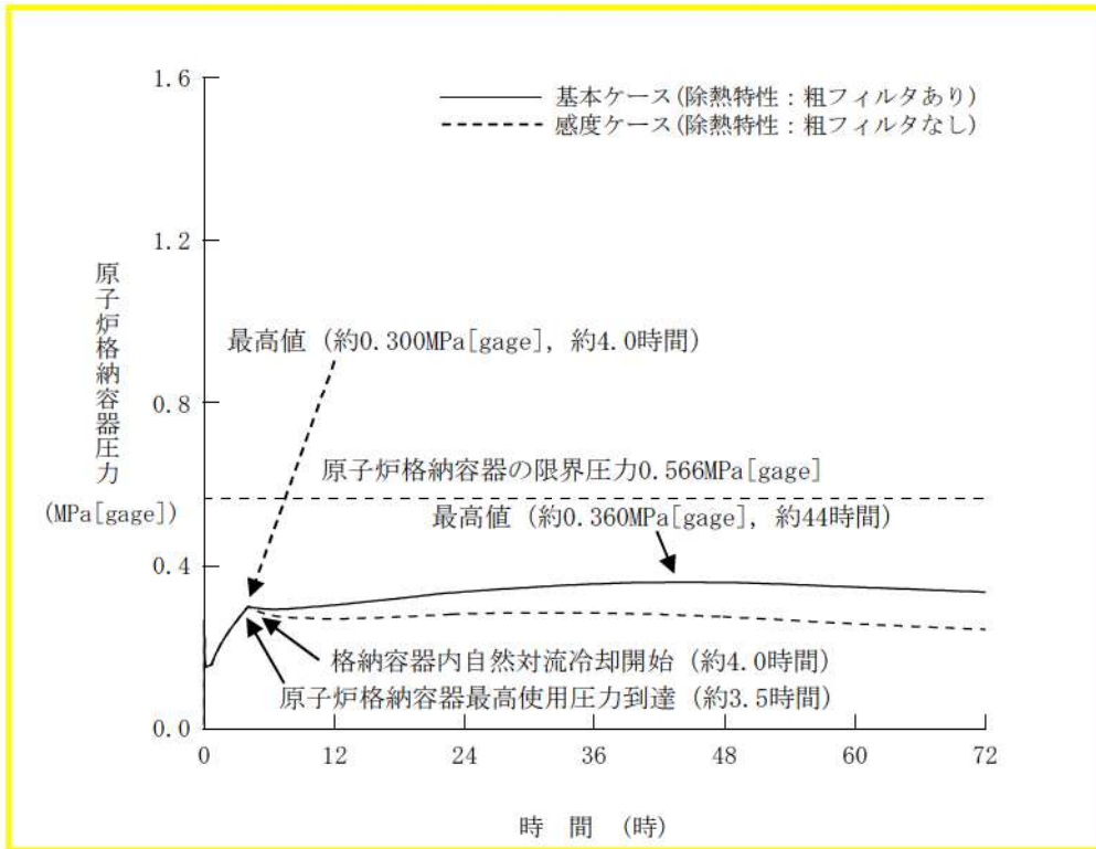
第 7.1.4.16 図 原子炉格納容器圧力の推移 (格納容器再循環ユニット除熱特性の影響確認)
