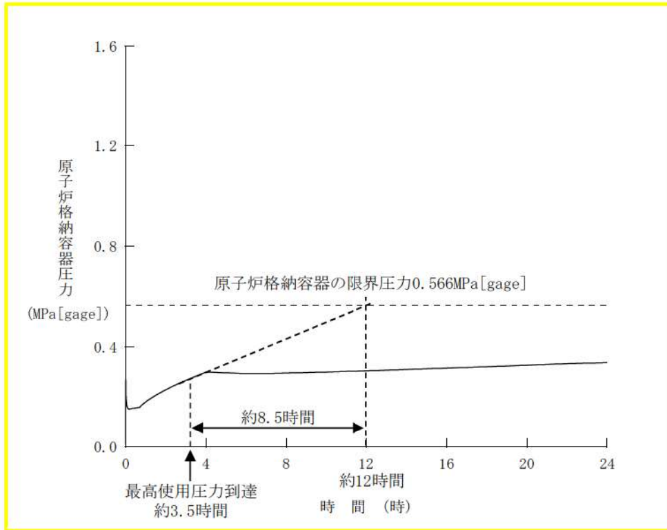
第 7.1.4.18 図 原子炉格納容器圧力の推移 (格納容器内自然対流冷却の操作時間余裕確認)
