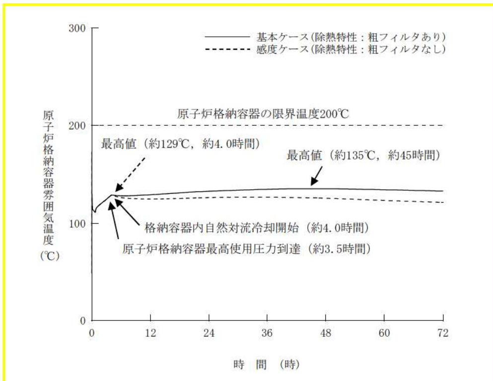
第 7.1.4.17 図 原子炉格納容器雰囲気温度の推移 (格納容器再循環ユニット除熱特性の影響確認)
