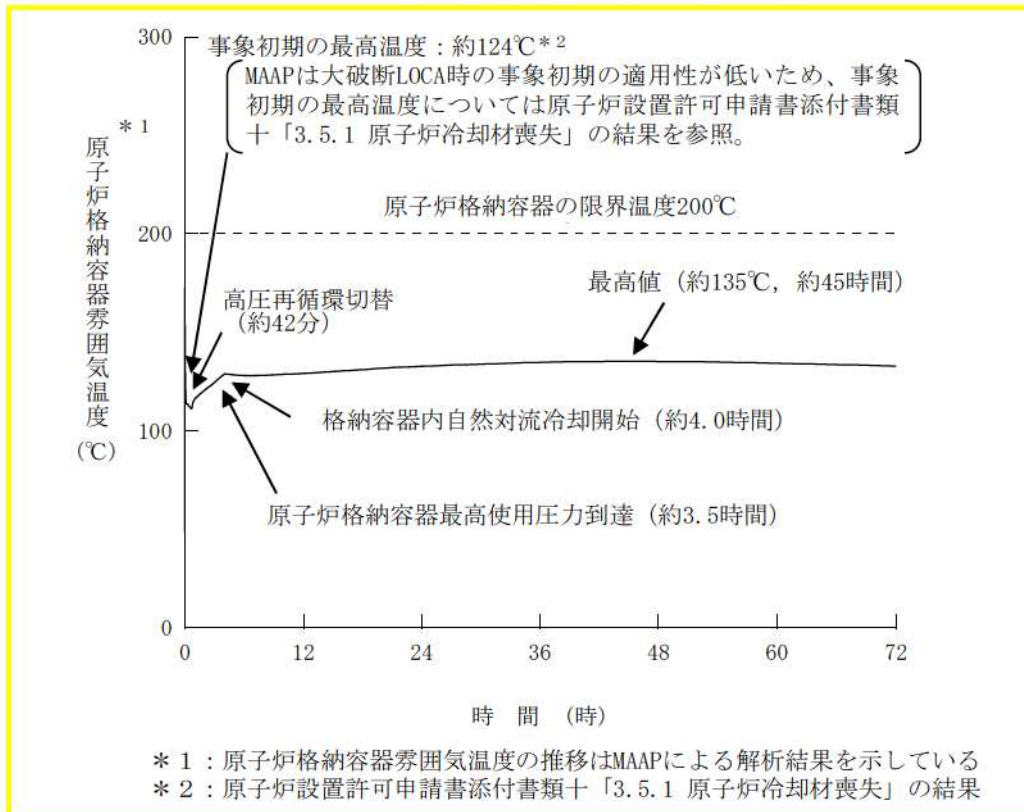
第 7.1.4.15 図 原子炉格納容器雰囲気温度の推移
