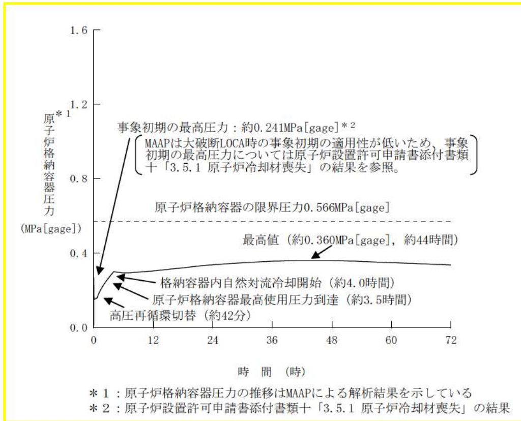
第 7.1.4.14 図 原子炉格納容器圧力の推移
