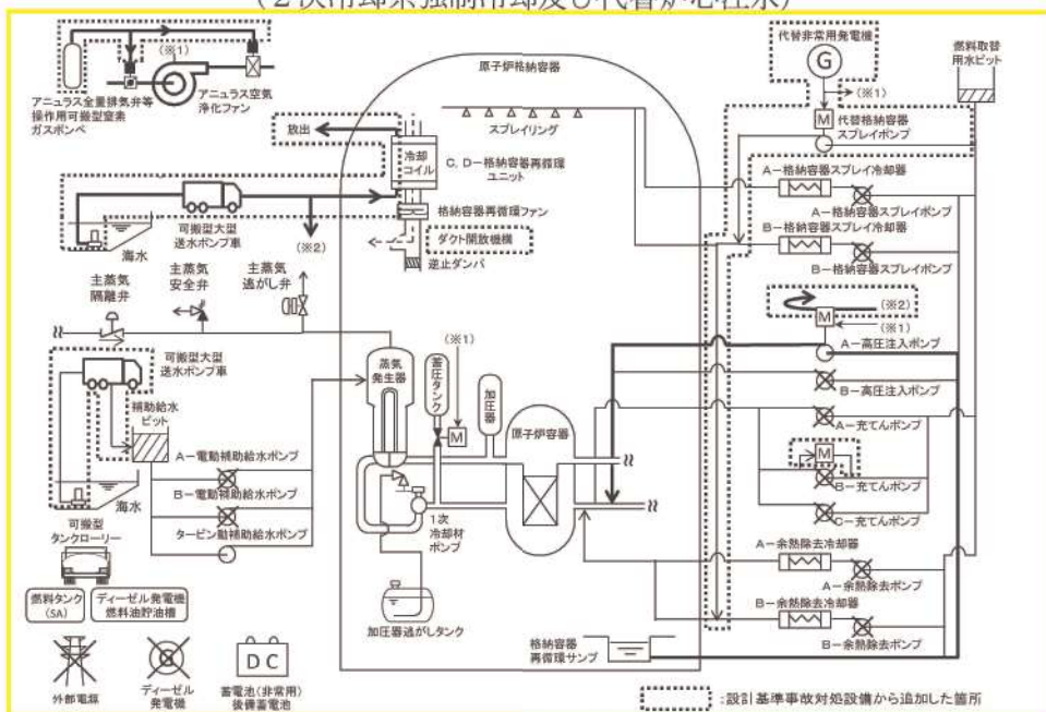
図2 「外部電源喪失時に非常用所内交流電源が喪失し、原子炉補機冷却機能の喪失及びRCPシールLOCAが発生する事故」の重大事故等対策の概略系統図 (格納容器内自然対流冷却及び高圧代替再循環)
