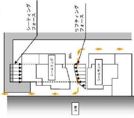
図1 No. 1シールの作動原理模式図
