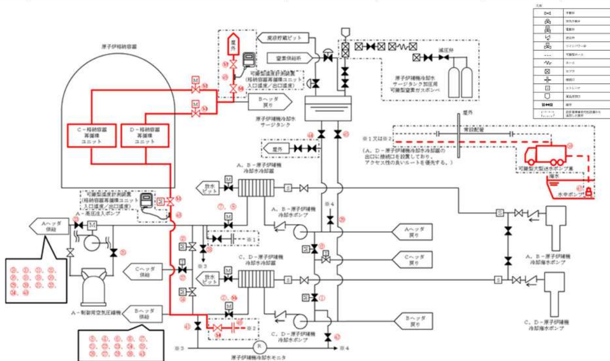
図 50-4-3 可搬型大型送水ポンプ車を用いたC, D-格納容器再循環ユニットによる格納容器内自然対流冷却
