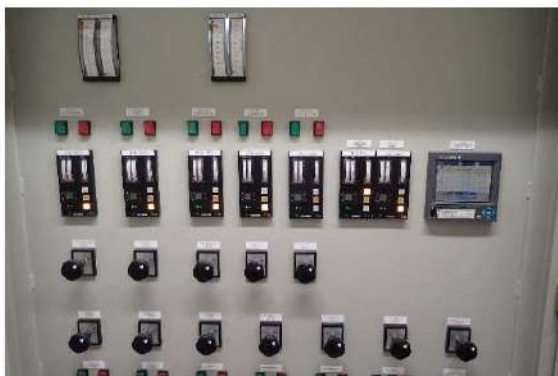
図3 中央制御室外原子炉停止盤における配置例
