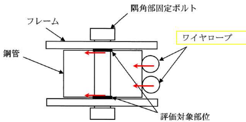
接続用の治具を構成する隅角固定ボルトの荷重状態
