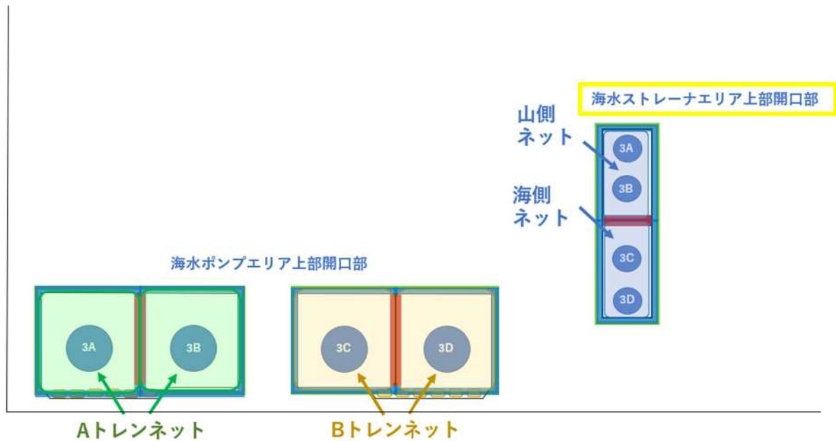
図3 竜巻防護ネット 平面図
