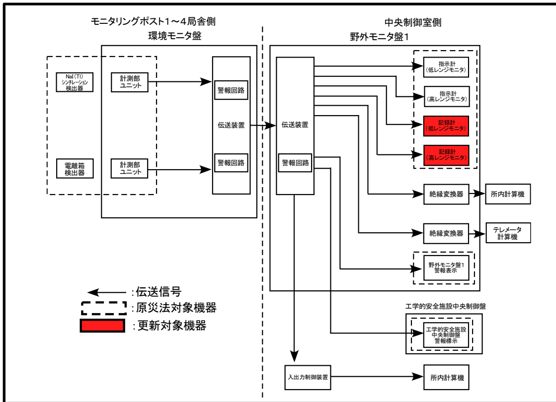
検査対象設備図(モニタリングポスト1, 2, 3, 4)
