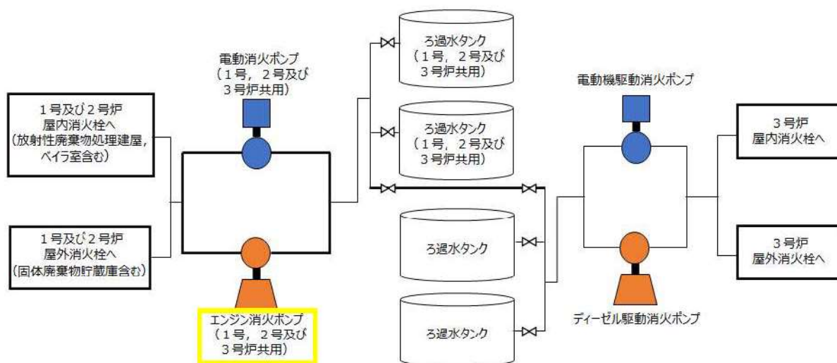
第41-1-14図：消火用水供給系の概要
