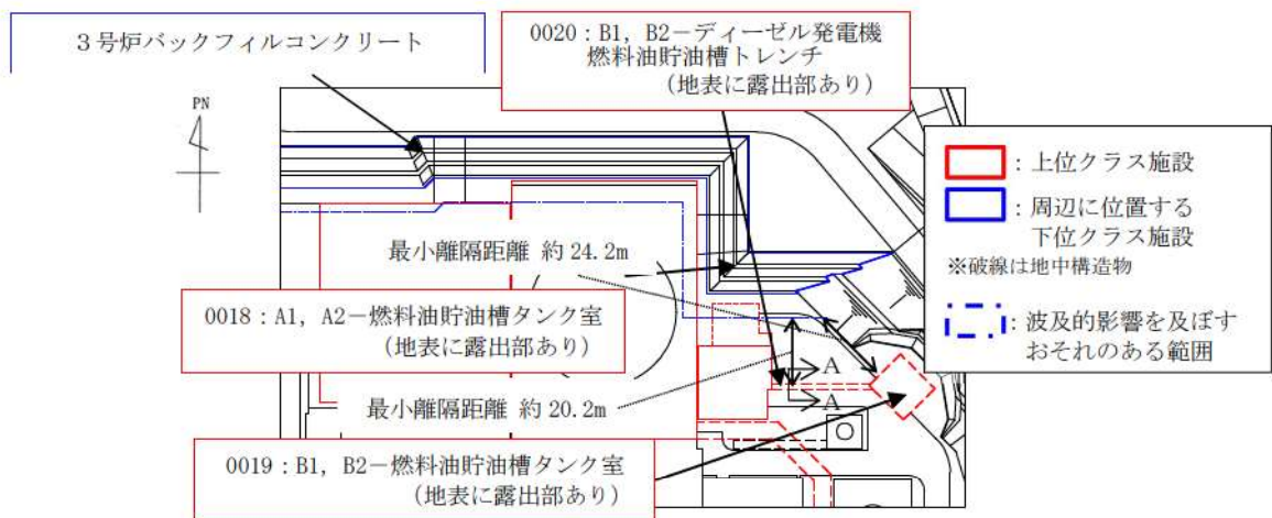
第4-11図 燃料油貯油槽タンク室周辺 平面図
