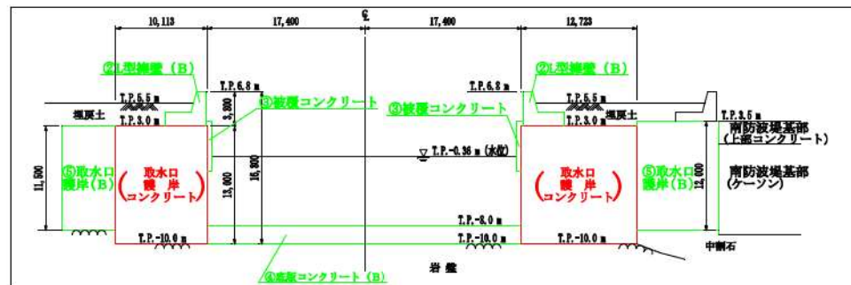
第4-3図 断面図（B-B断面）
