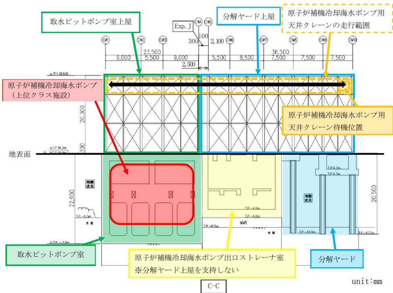
第 1-2 図 概略断面図 (2/2)
