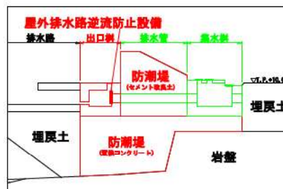
第6.1-3図 防潮堤 断面図 (A-A断面)
