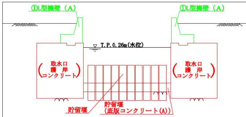
第6.1-9図 貯留堰周辺 断面図
