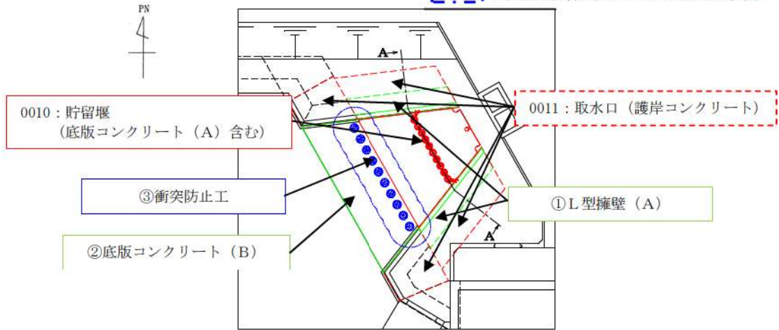
第6.1-8図 貯留堰周辺 平面図
