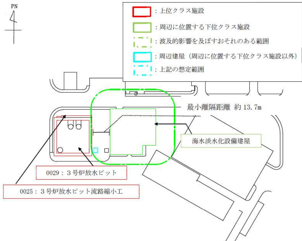
第6.1-10図 3号炉放水ピット流路縮小工周辺 平面図
