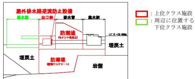
第 6.1-4 図 屋外排水路逆流防止設備 縦断面図
