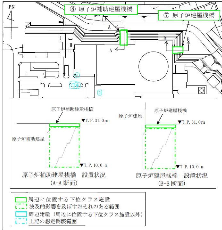
第 3.3-8 図 上位クラス施設に対する波及影響を及ぼすおそれのある範囲 (原子炉建屋棧橋, 原子炉補助建屋棧橋)
