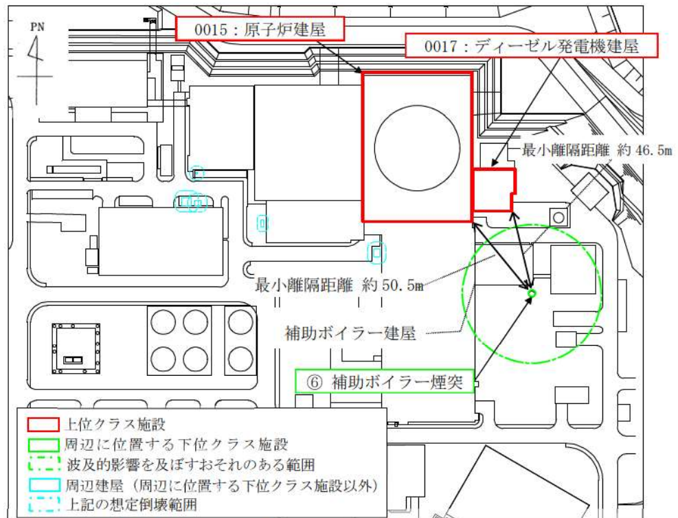
第 3.3-7 図 上位クラス施設に対する波及的影響を及ぼすおそれのある範囲（補助ボイラー煙突）
