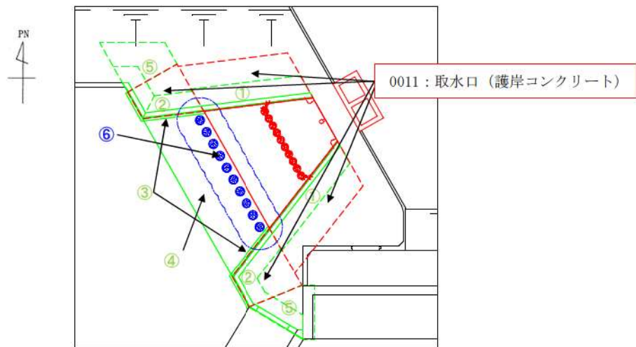
第 4-1 図 取水口周辺 平面図
