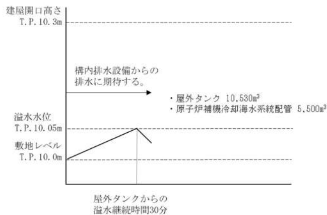
図 2 地震発生後の溢水水位イメージ
