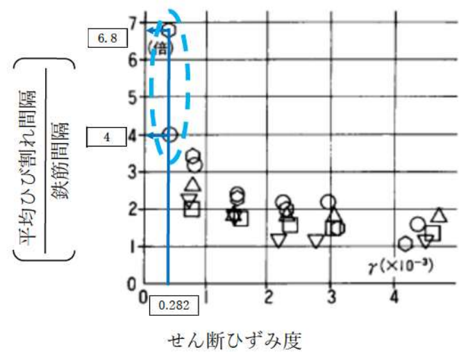
図 9 平均ひび割れ間隔／鉄筋間隔
