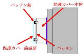
図2 現場での被水状況を考慮した被水対策について
