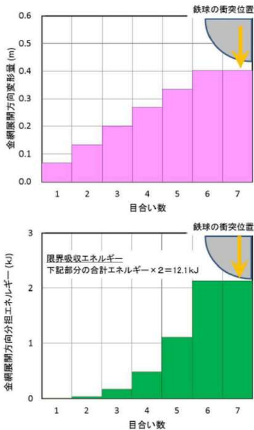
図2 予備試験結果と吸収エネルギー評価式との比較
