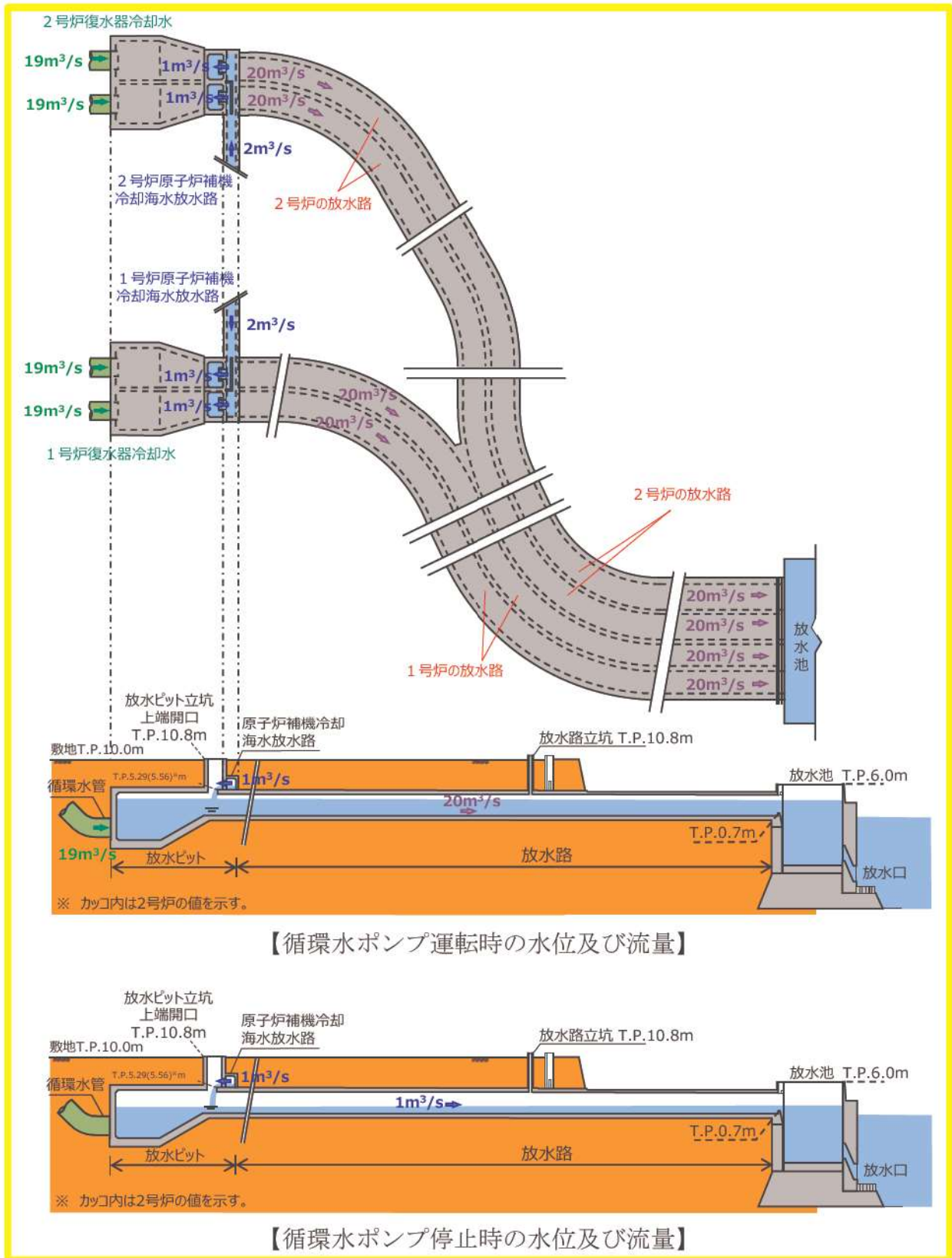
図6 1号及び2号炉放水系概要
