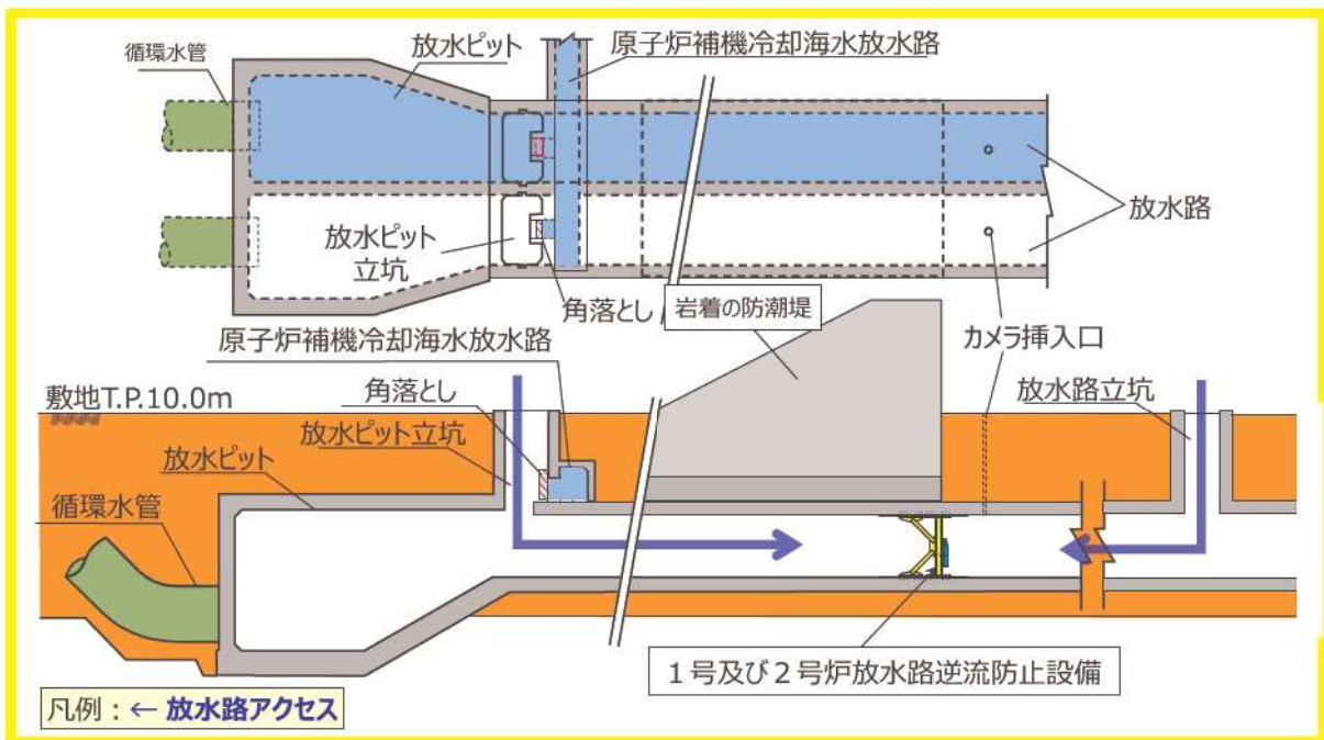
図 13 逆流防止設備設置後の施設管理
