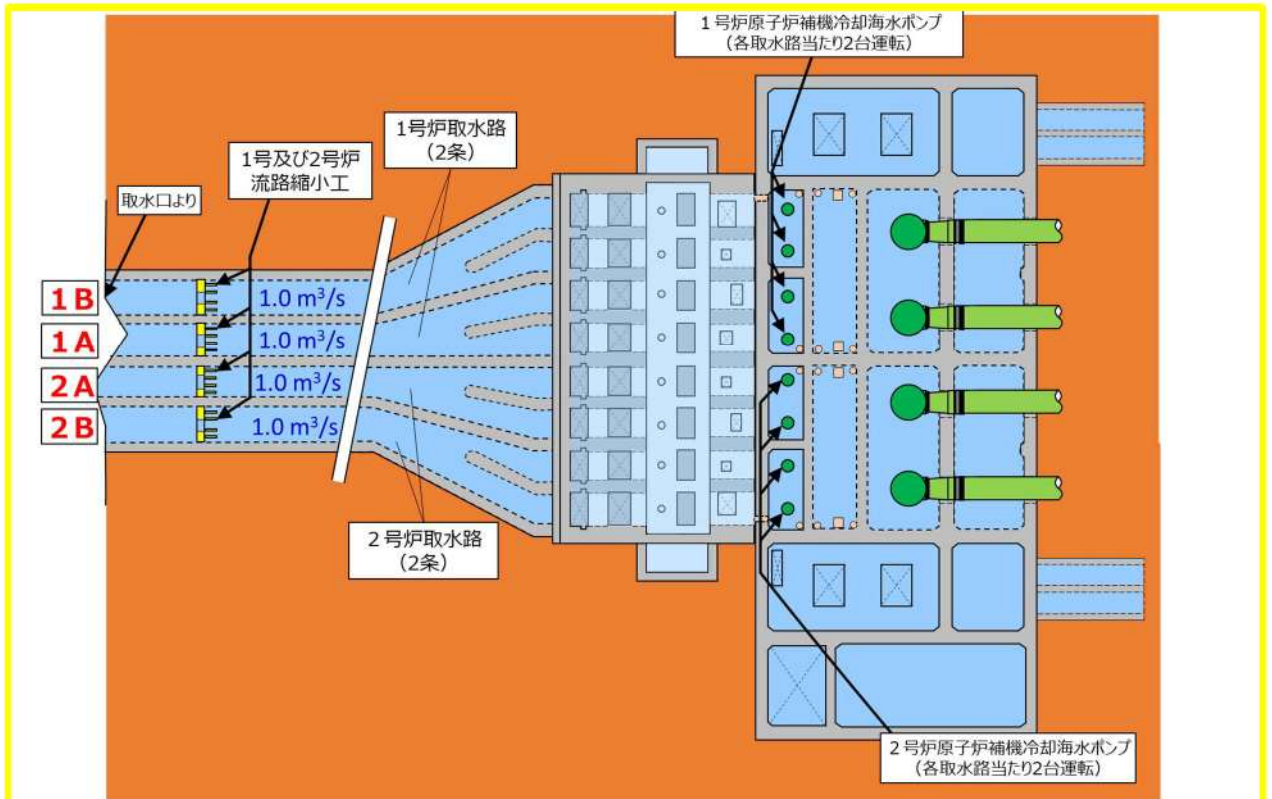
図5 取水路の流量を示す平面図
