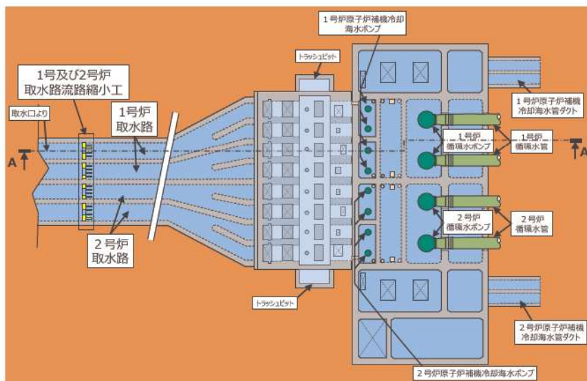
【平面図】
