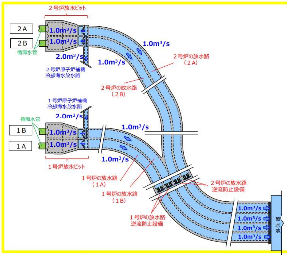
図9 放水路の流量を示す平面図
