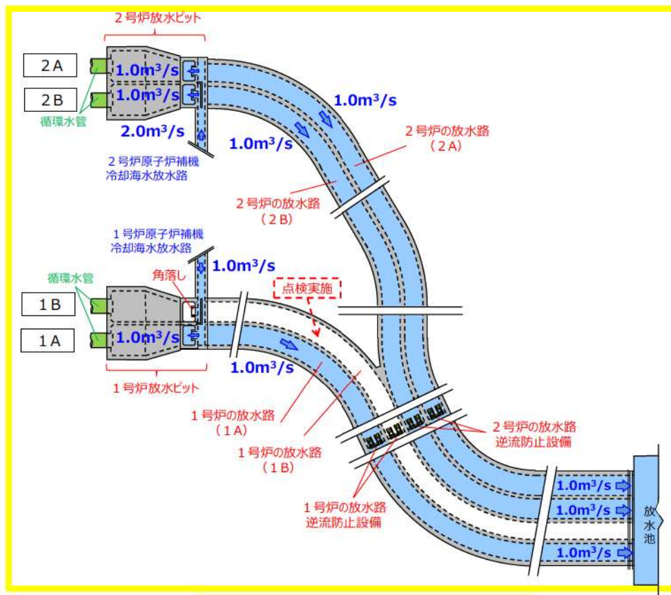
図10 放水路の流量を示す平面図
