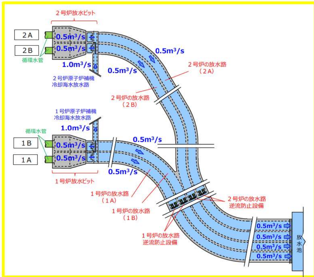
図7 放水路の流量を示す平面図
