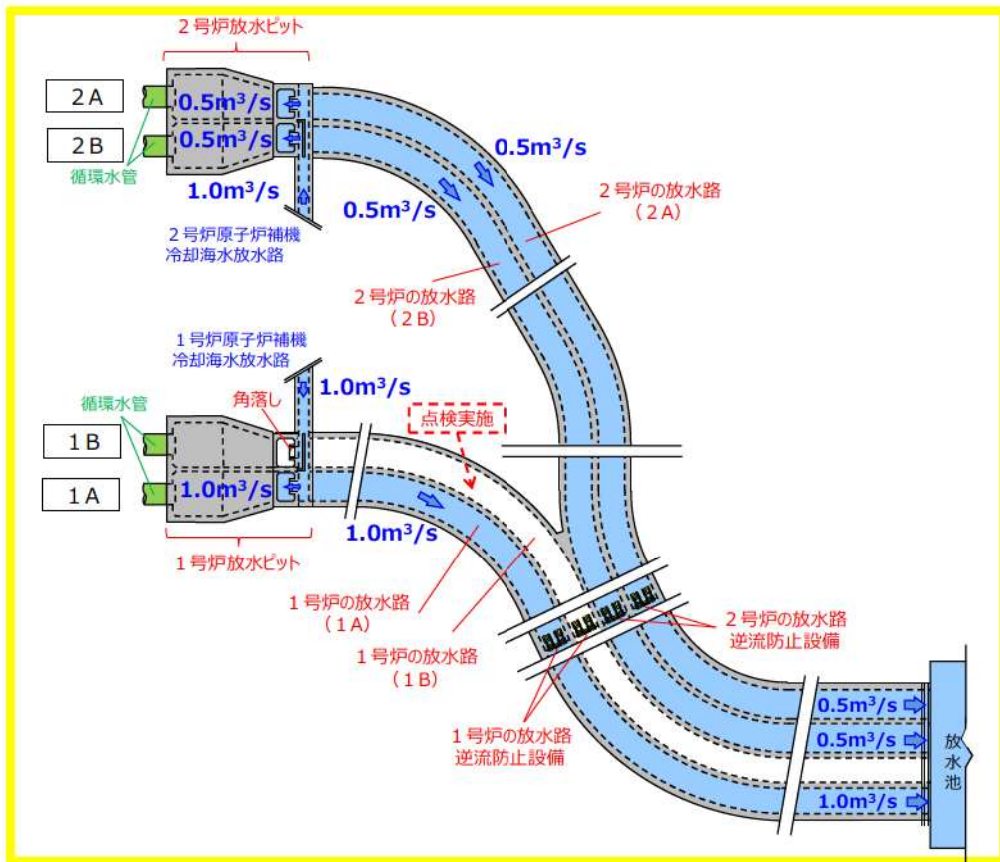
図8 放水路の流量を示す平面図
