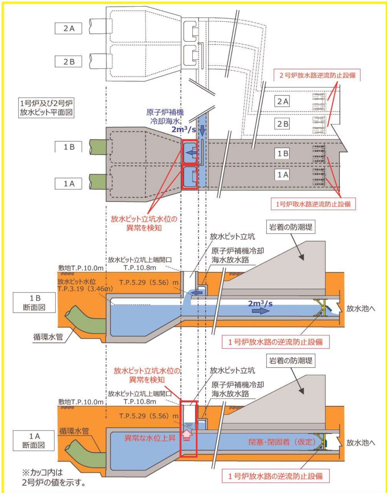
図 12 逆流防止設備の異常の検知位置（1号炉で発生した場合）
