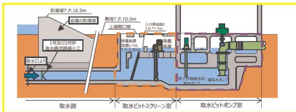
【A-A断面図】
