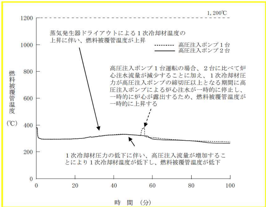
図6 燃料被覆管温度の推移
