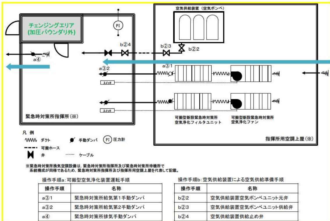
第1.18.3図 可搬型空気浄化装置運転及び空気供給装置(空気ボンベ)準備の概略系統図
