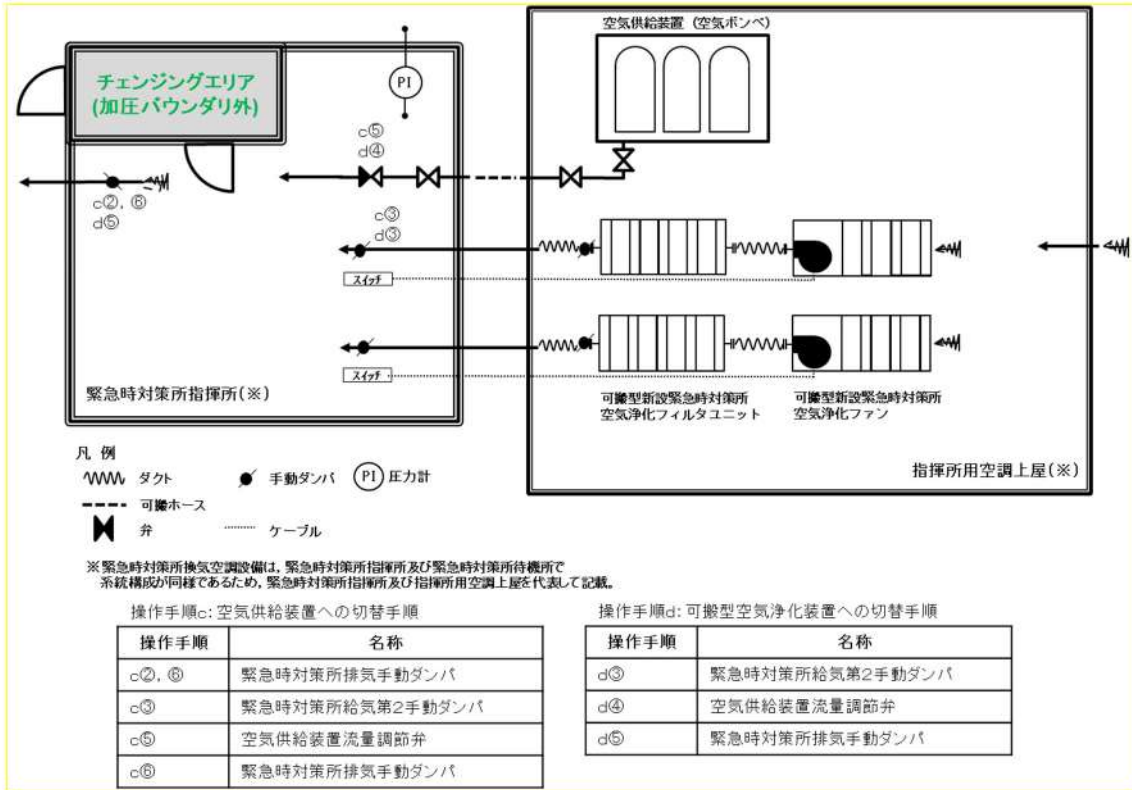
第1.18.9図 緊急時対策所換気空調設備系統概略図
