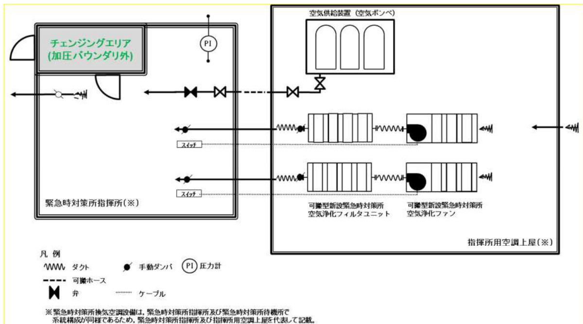
第1. 18. 23図 空気供給装置 (空気ポンベ) による空気供給準備概要図
