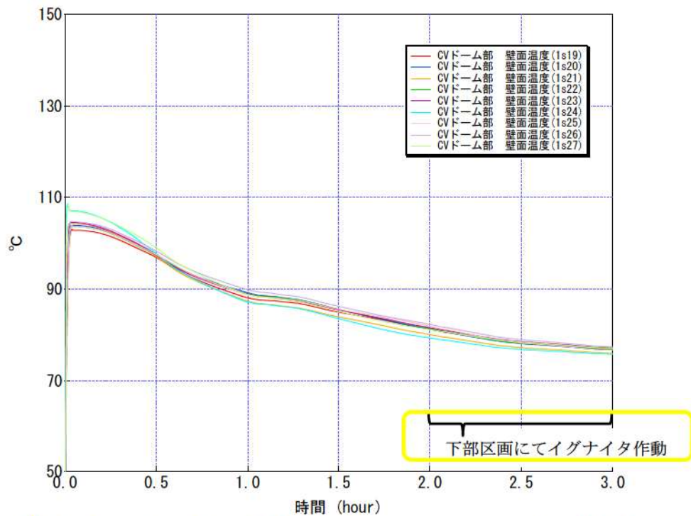
別図 1 4 イグナイタ着火時のドーム部頂部の壁面温度変化 (拡大) 泊 3 号炉 GOTHIC 解析「大破断 LOCA+ECCS 注入失敗 (Zr-水反応割合 81%)」
