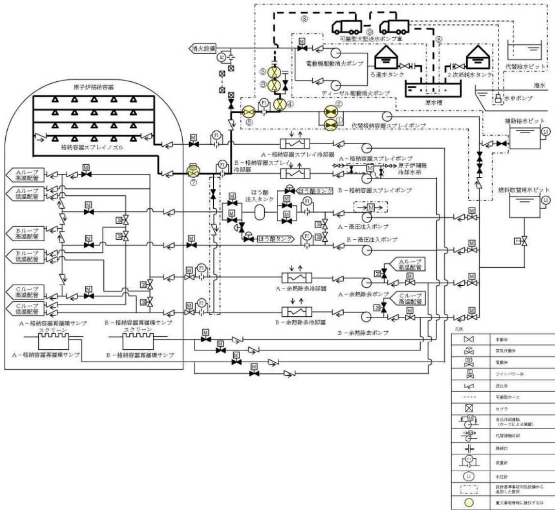
図 49-10-4 原水槽を水源とした可搬型大型送水ポンプ車による原子炉格納容器内へのスプレィの概要図
