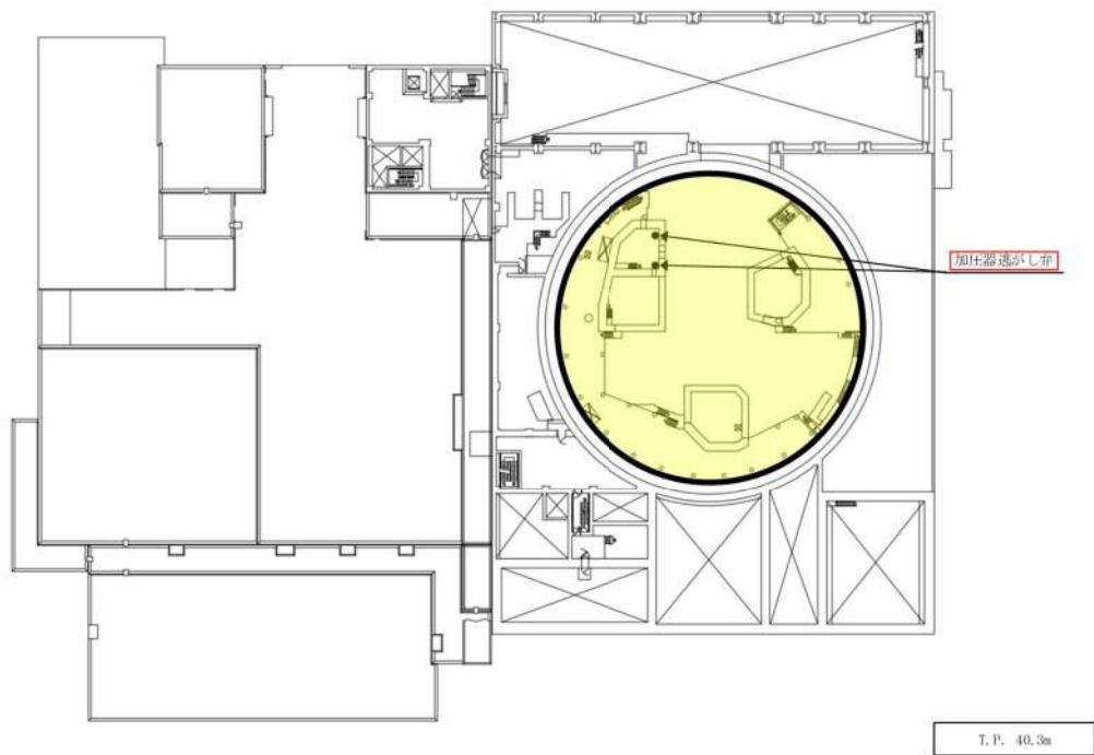
第13図 1次系のフィードアンドブリード（高圧注入ポンプ）に関する機器の配置（3／3）
