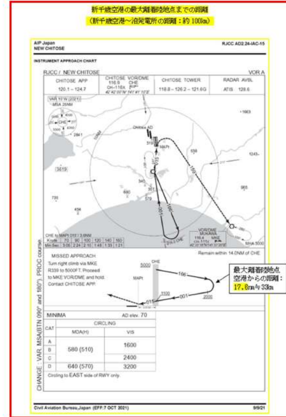
図2 新千歳空港の最大離着陸地点
