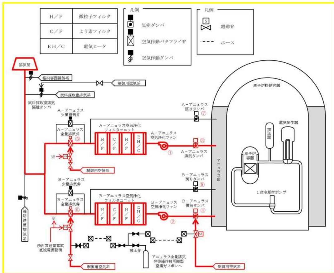
図 59-4-3 アニュラス空気浄化設備 系統概要図(全交流動力電源及び直流電源が健全である場合)
