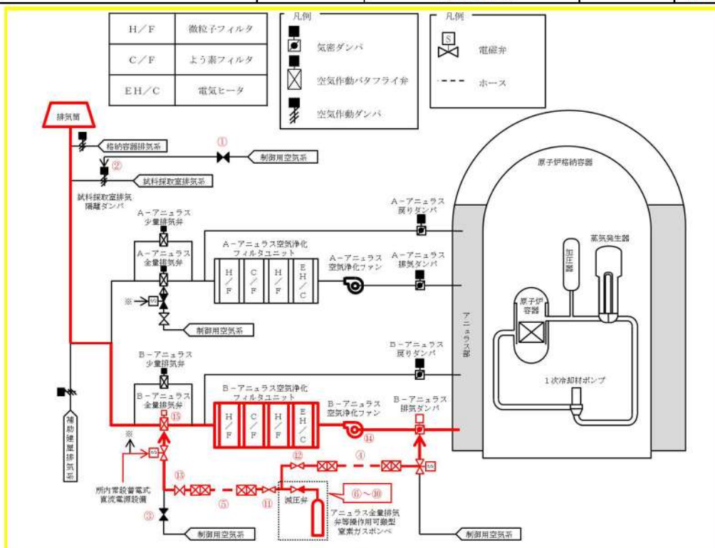
図 59-4-4 アニュラス空気浄化設備 系統概要図 (全交流動力電源及び直流電源喪失した場合)
