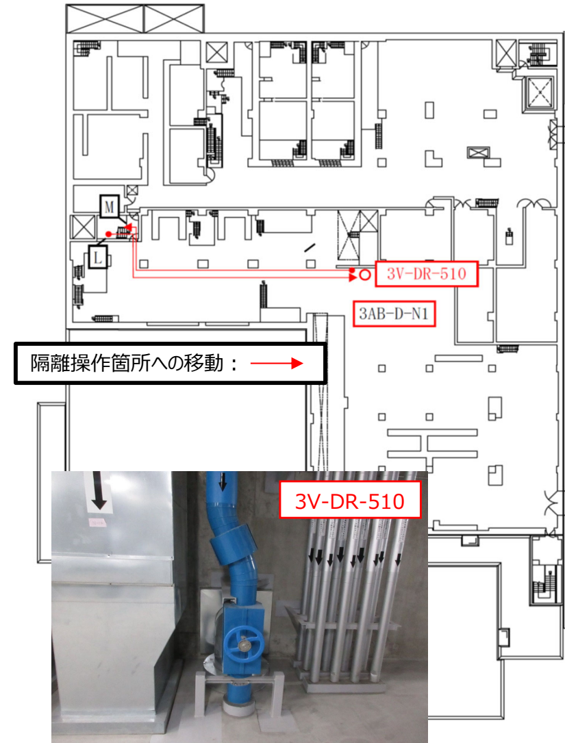
原子炉補助建屋 T.P.24.8m
