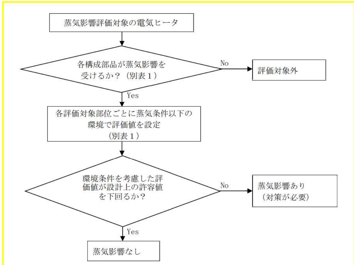
図1 電気ヒータの耐蒸気性能評価フロー
