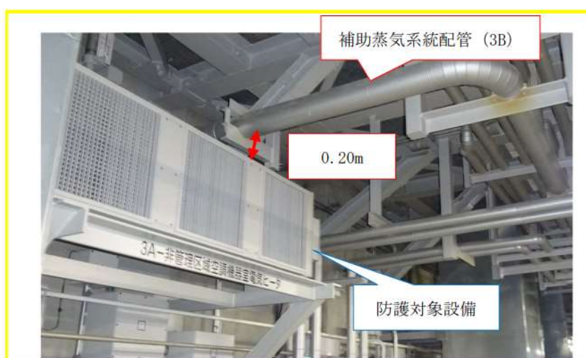
図 1 補助蒸気系統配管と 3 A-非管理区域空調機器室電気ヒータとの位置関係
