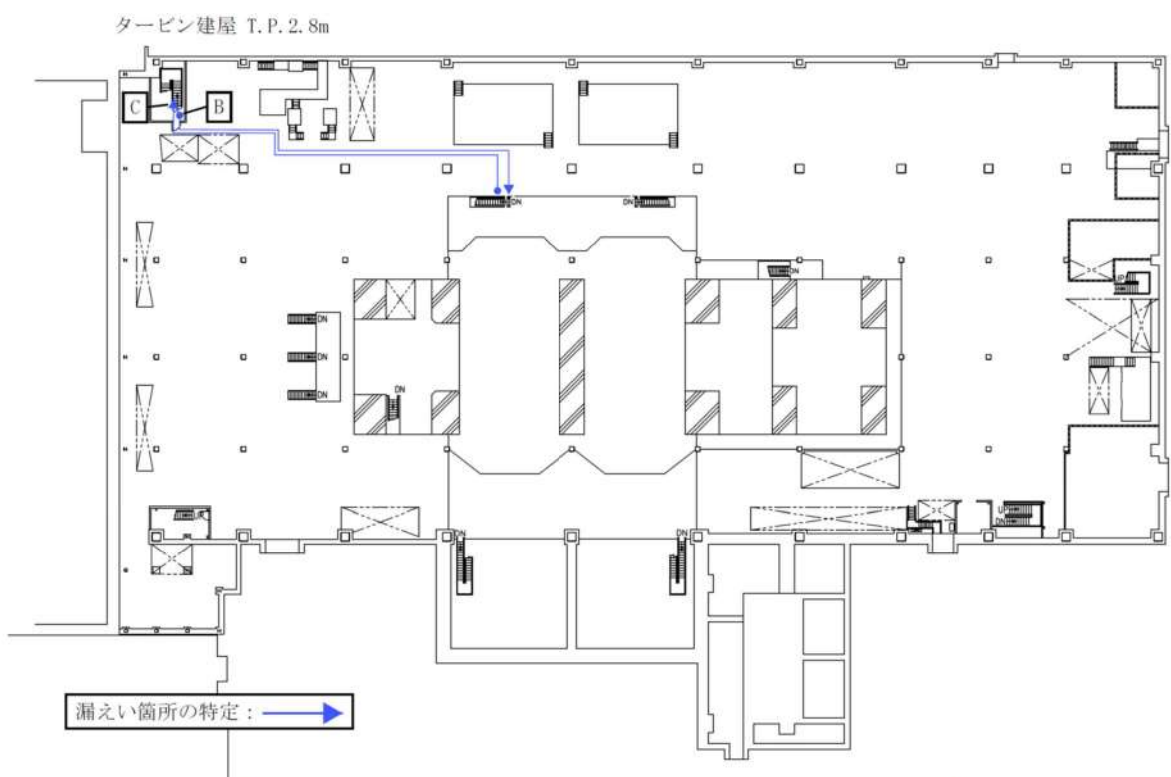
図 2 地震時の隔離操作時におけるアクセス通路 (2/14)
