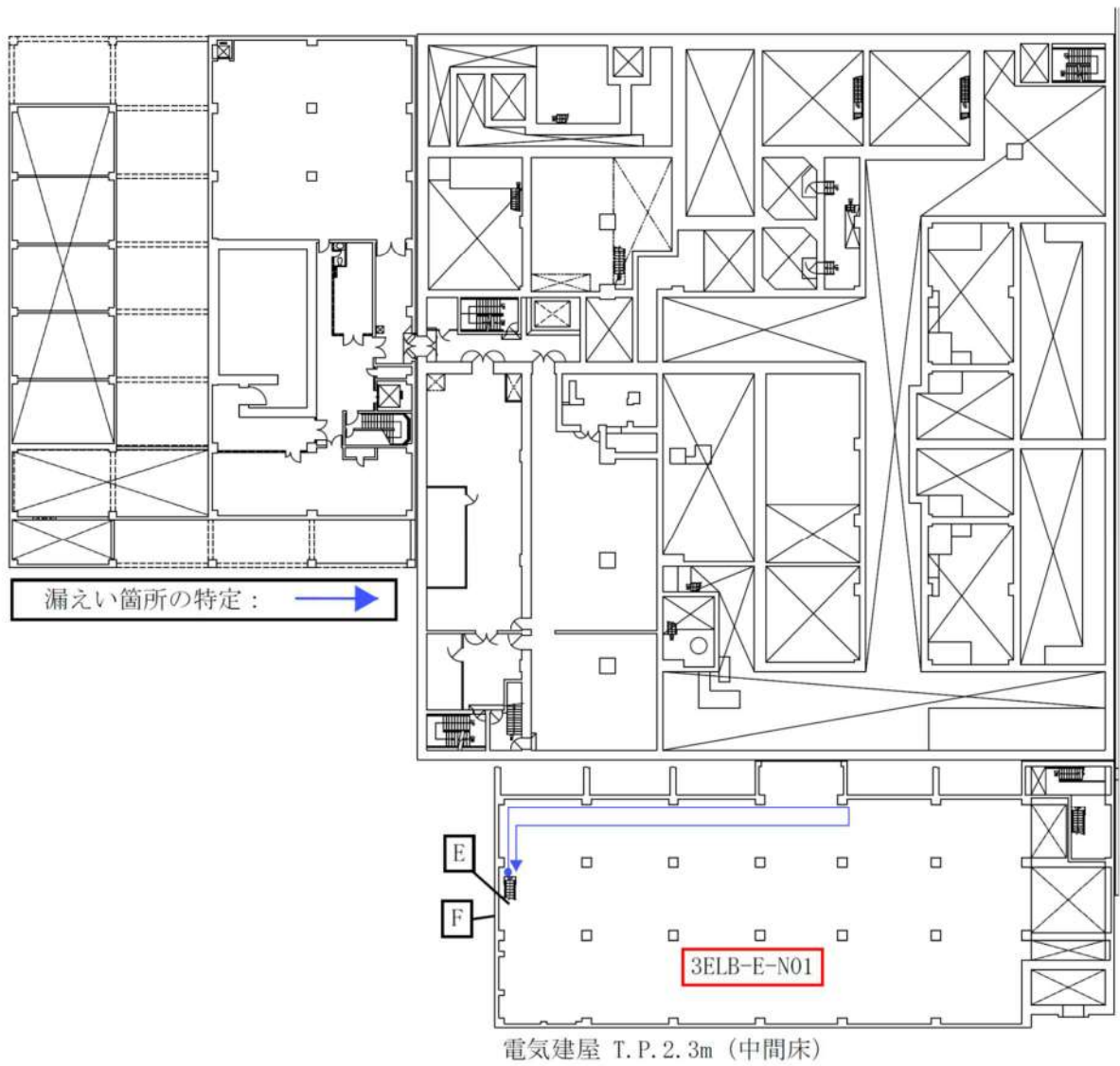
図2 地震時の隔離操作時におけるアクセス通路 (5/14)
