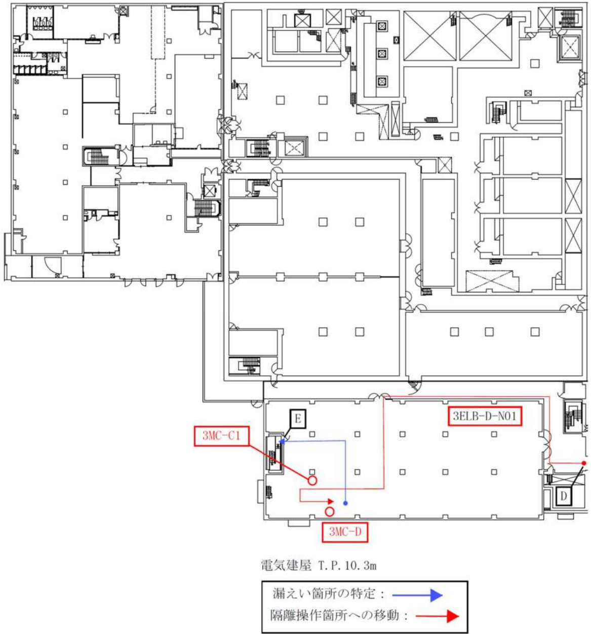
図2 地震時の隔離操作時におけるアクセス通路 (4/14)
