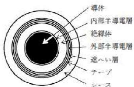
(高圧動力ケーブルの例)
