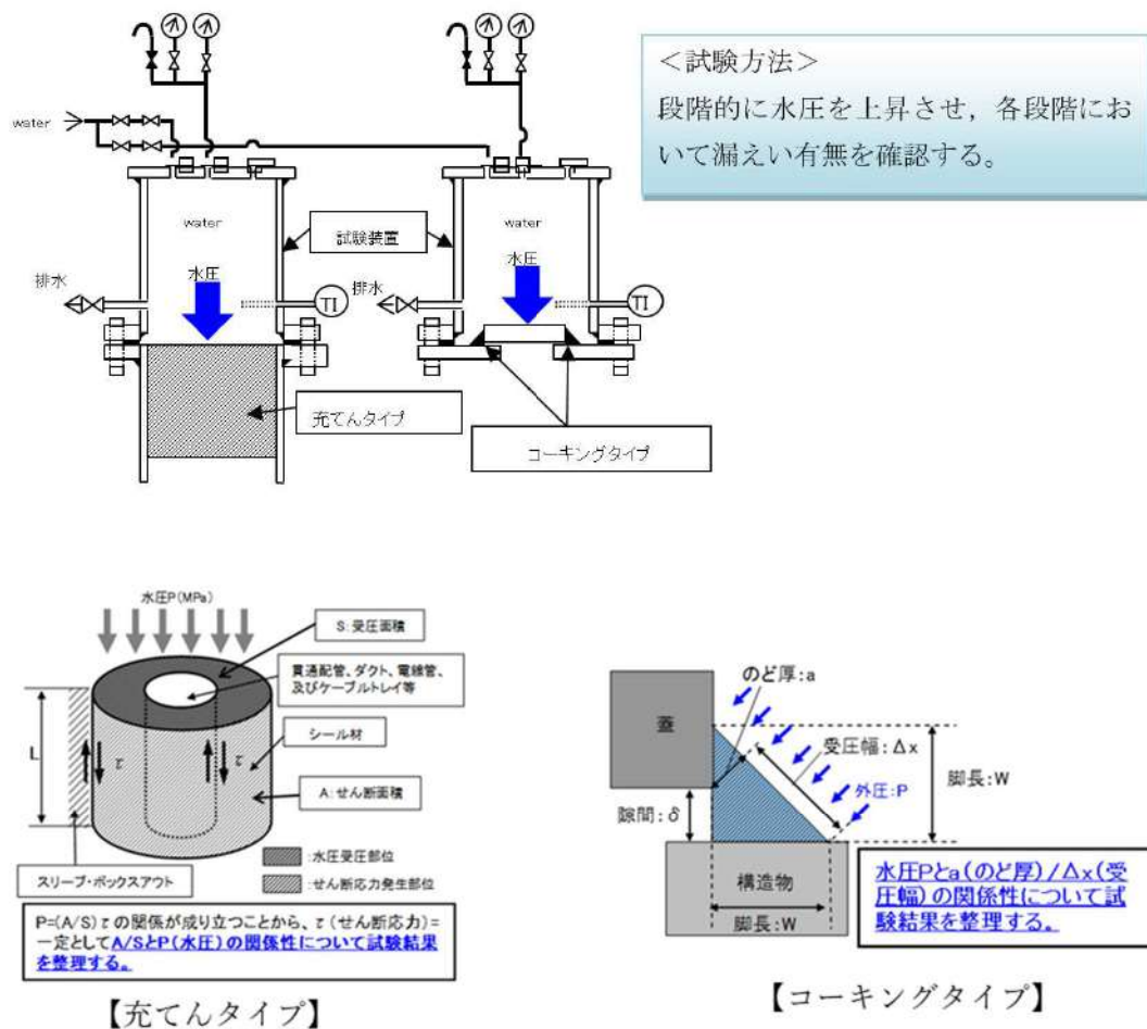
図 9 シリコンシーラント及び充てんシーラントの耐水圧試験概要図
