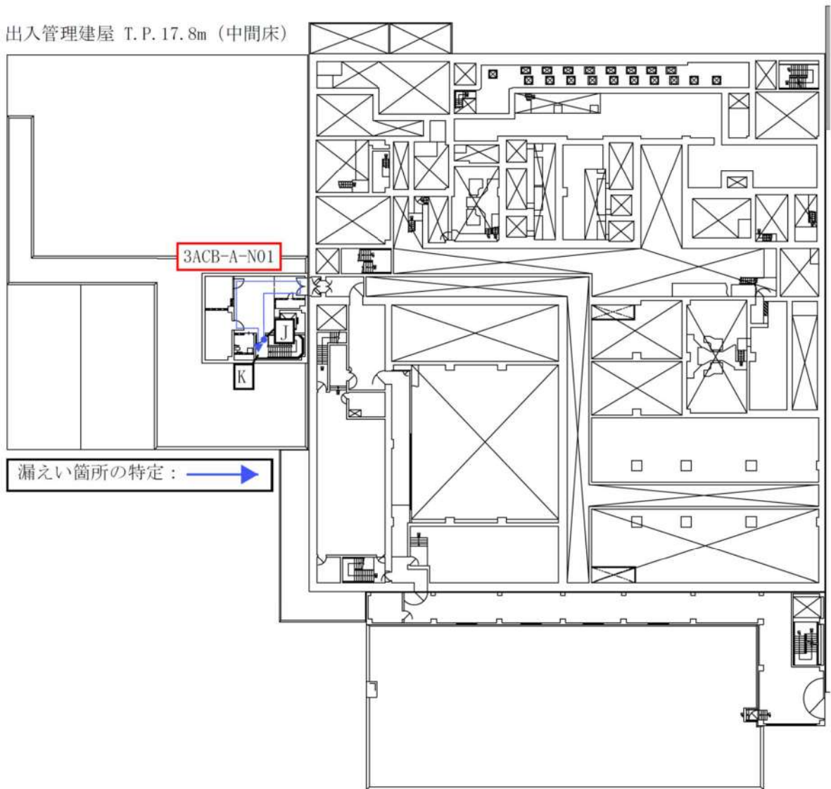
図 2 地震時の隔離操作時におけるアクセス通路 (10/14)
