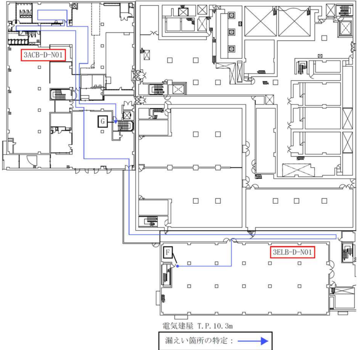
図2 地震時の隔離操作時におけるアクセス通路 (6/14)
