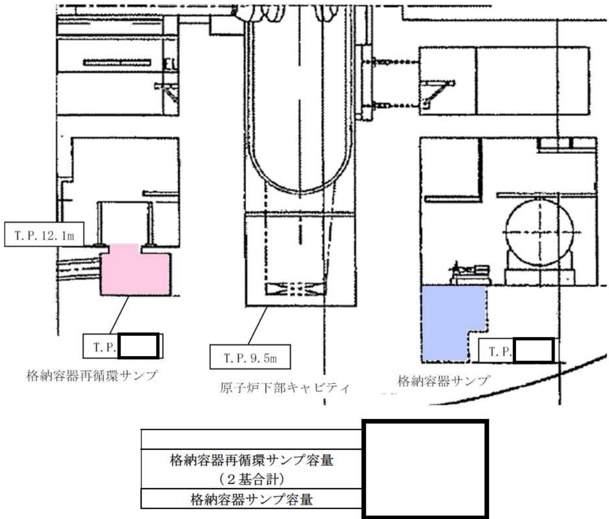
図9 原子炉格納容器内断面図
