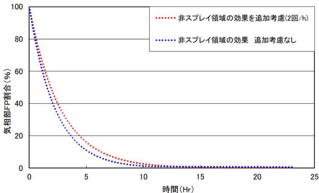
図1 スプレイ除去効果の比較
