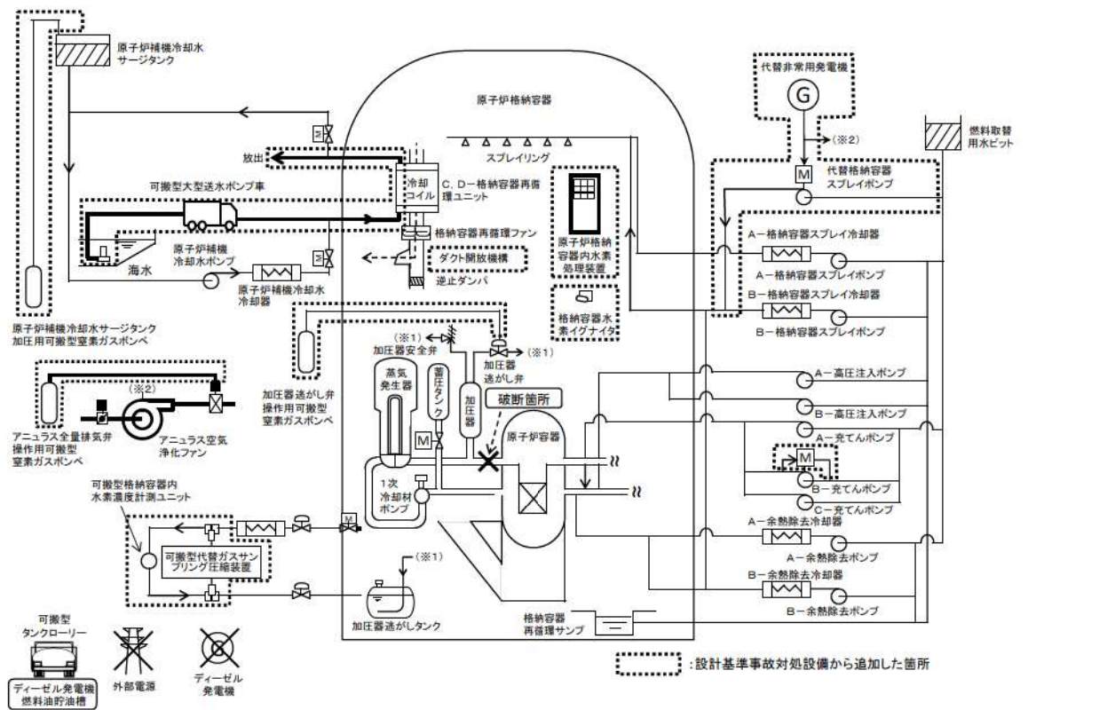
第 7.2.1.1.1 図 「雰囲気圧力・温度による静的負荷（格納容器過圧破損）」 の重大事故等対策の概略系統図（2 / 2）（格納容器内自然対流冷却）
