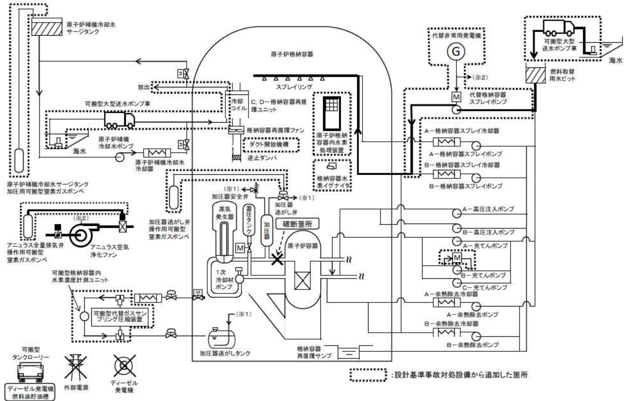
第 7.2.1.1.1 図 「雰囲気圧力・温度による静的負荷（格納容器過圧破損）」 の重大事故等対策の概略系統図（1 / 2）（代替格納容器スプレイ）
