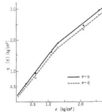
図-3 B_{0.44}^{0.84} 砂の \sigma-\tau_f と \sigma-\tau_f' 関係図
