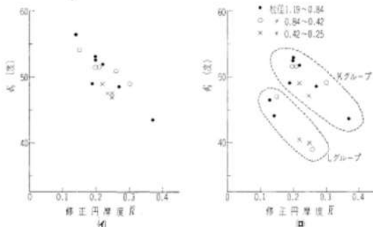
図-8 \phi , \phi' と修正円摩度 R との関係図
