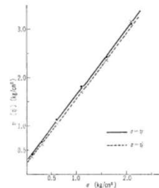
図-4 C_{0.44}^{0.84} 砂の \sigma-\tau_f と \sigma-\tau_f' 関係図
