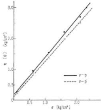
図-6 H_{0.84}^{1.19} 砂の \sigma - \tau と \sigma - \tau' 関係図
