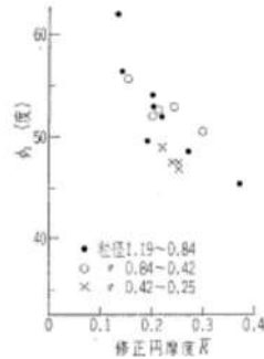
図-7 \phi_w と修正円摩度 \bar{R} との関係
