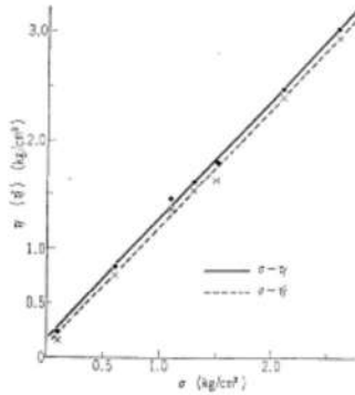
図-5 G_{0.25}^{0.84} 砂の \sigma - \tau と \sigma - \tau' 関係図
