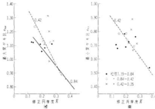
図-11 最大間ゲキ比, 最小間ゲキ比と修正円率指数との関係図
