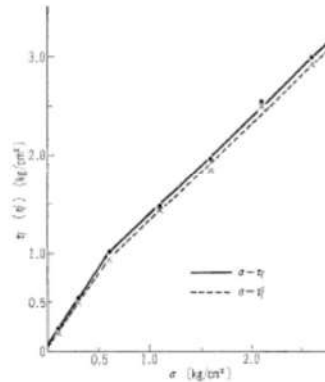
図-2 A_{0.44}^{1.19} 砂の \sigma-\tau_f と \sigma-\tau_f' 関係図
