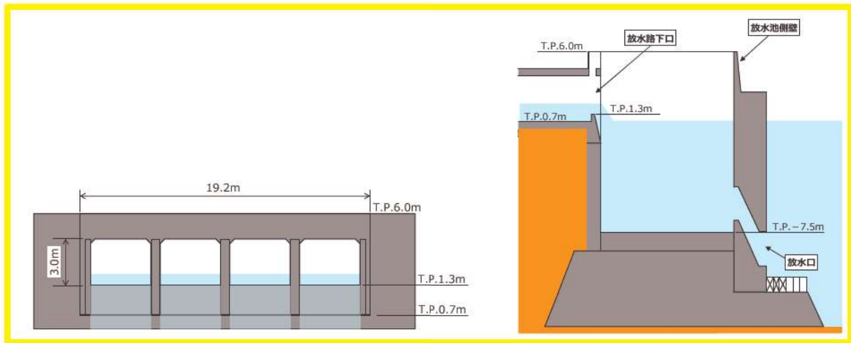
【1号及び2号炉放水路下口正面図】
