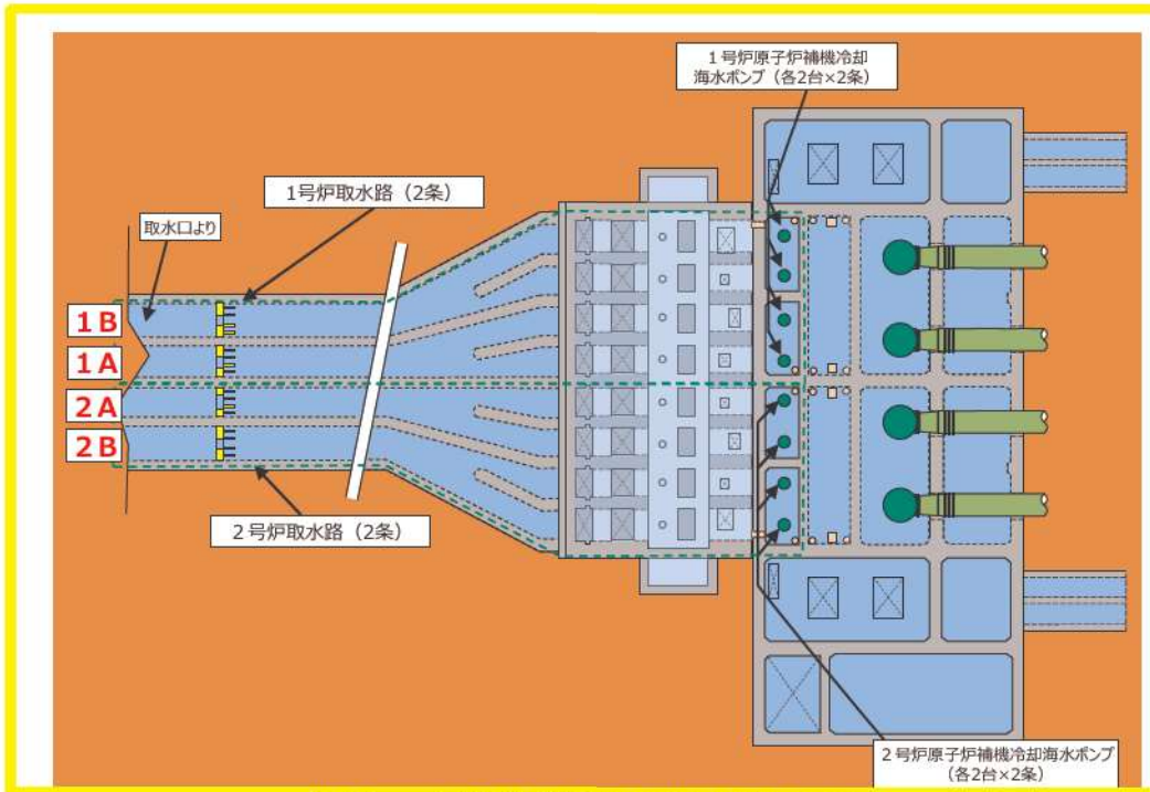
図3 1号及び2号炉取水路平面図
