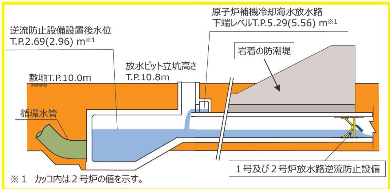
図4 1号及び2号炉放水系断面図
