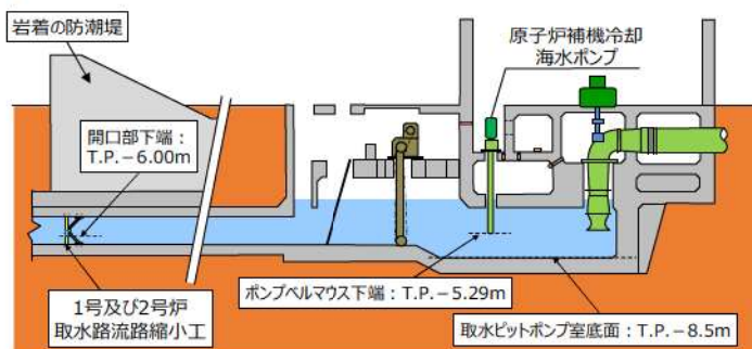
図5 1号及び2号炉取水系 断面 (ポンプベルマウス下端)
