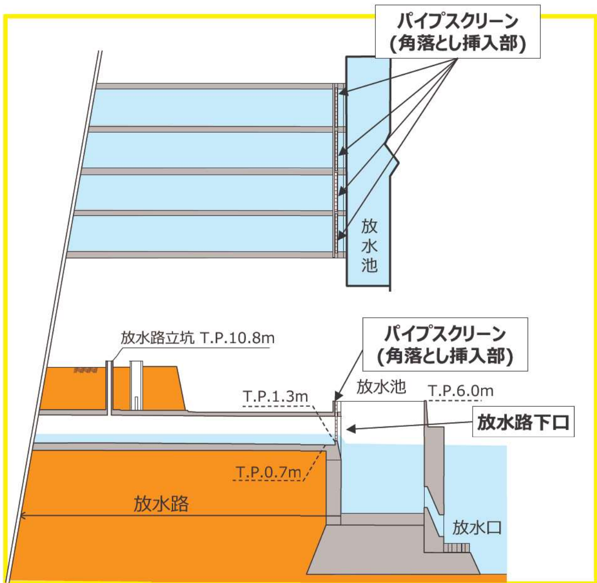
図8 パイプスクリーン計画
