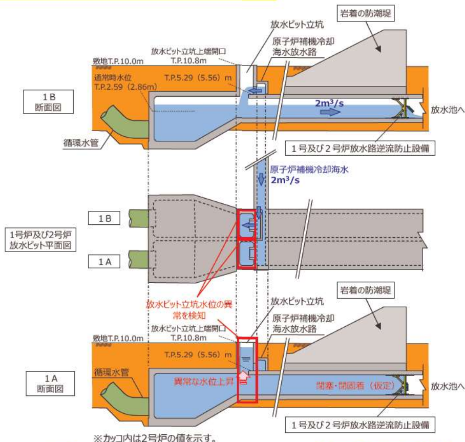
図 10 逆流防止設備の異常の検知位置 (1号炉の場合)
