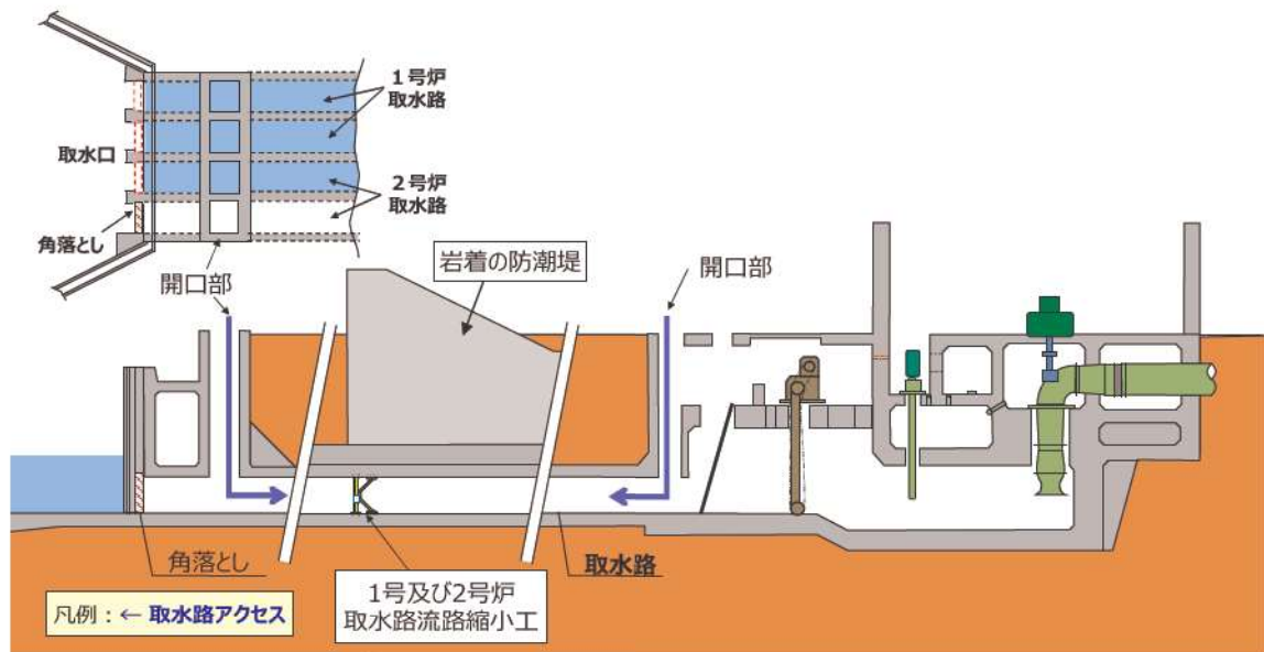
図9 流路縮小工設置後の施設管理
