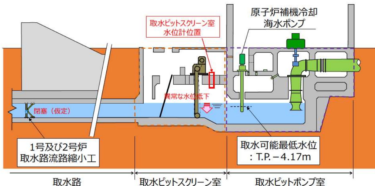
図10 流路縮小工の異常の検知位置
