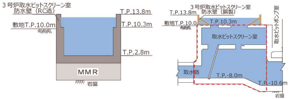
【B-B断面】
