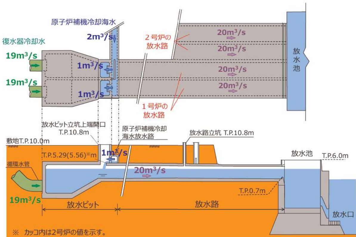
図3 1号及び2号炉放水系概要
