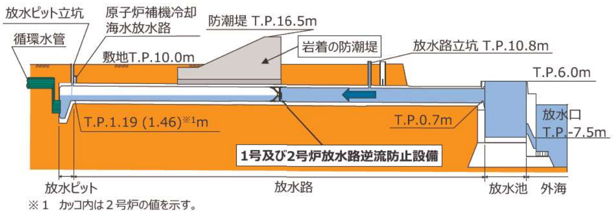
【1号及び2号炉放水系断面図】
