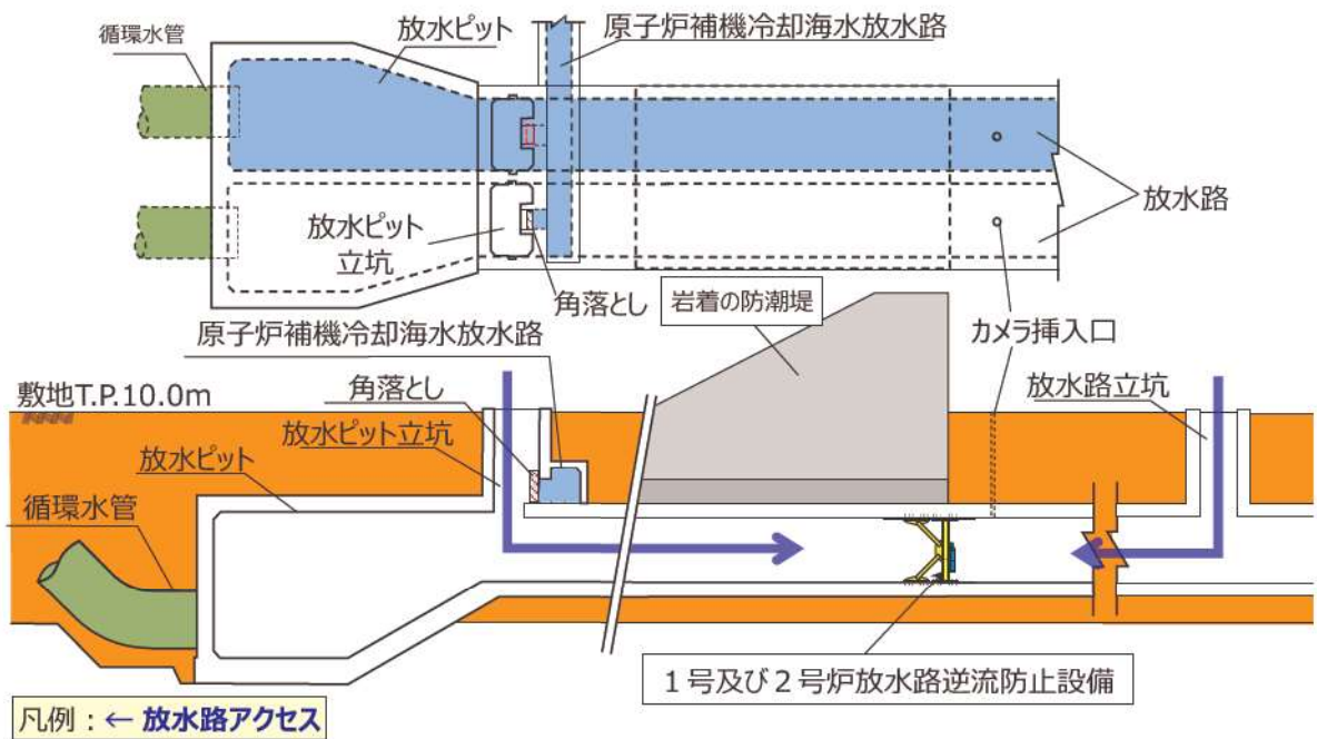
図9 逆流防止設備設置後の施設管理
