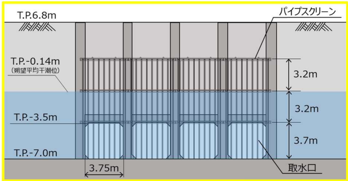
図8 通常時における1号及び2号炉取水口と海水面の関係
