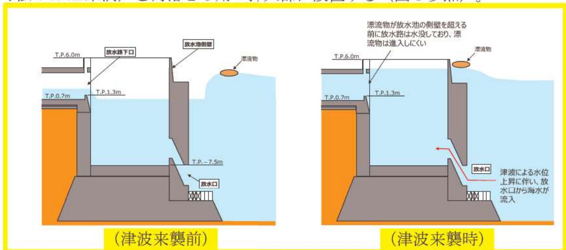
図7 放水池への津波到達時の1号及び2号炉放水路水位概要図
