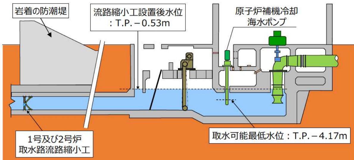
図4 1号及び2号炉取水系断面 (ポンプ取水可能最低水位)
