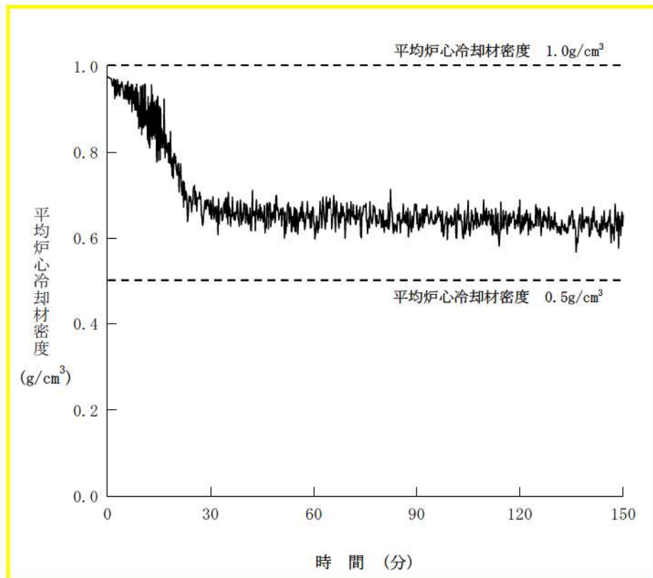
図3 原子炉冷却材の流出時の平均炉心冷却材密度の推移
