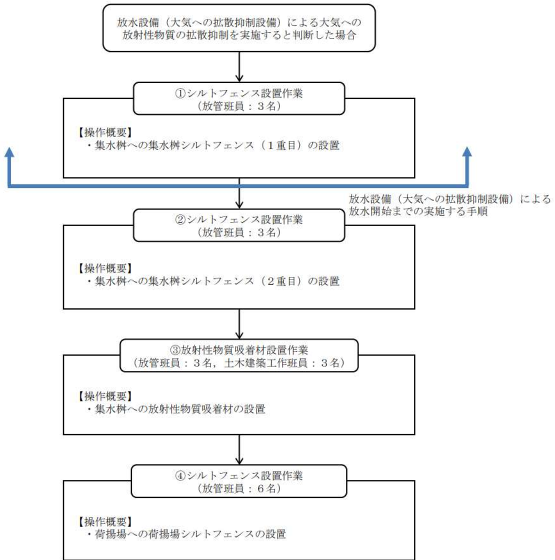
第 1.12.9 図 海洋への放射性物質の拡散手順の流れ
