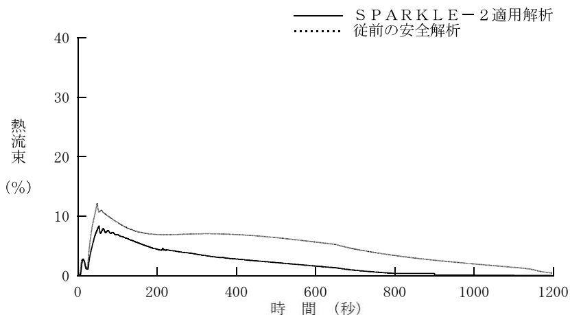
「主蒸気管破断」解析結果（熱流束）
