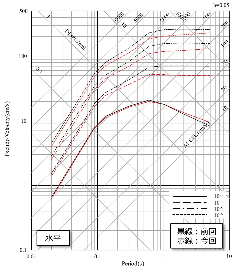
一様ハザードスペクトルの比較
