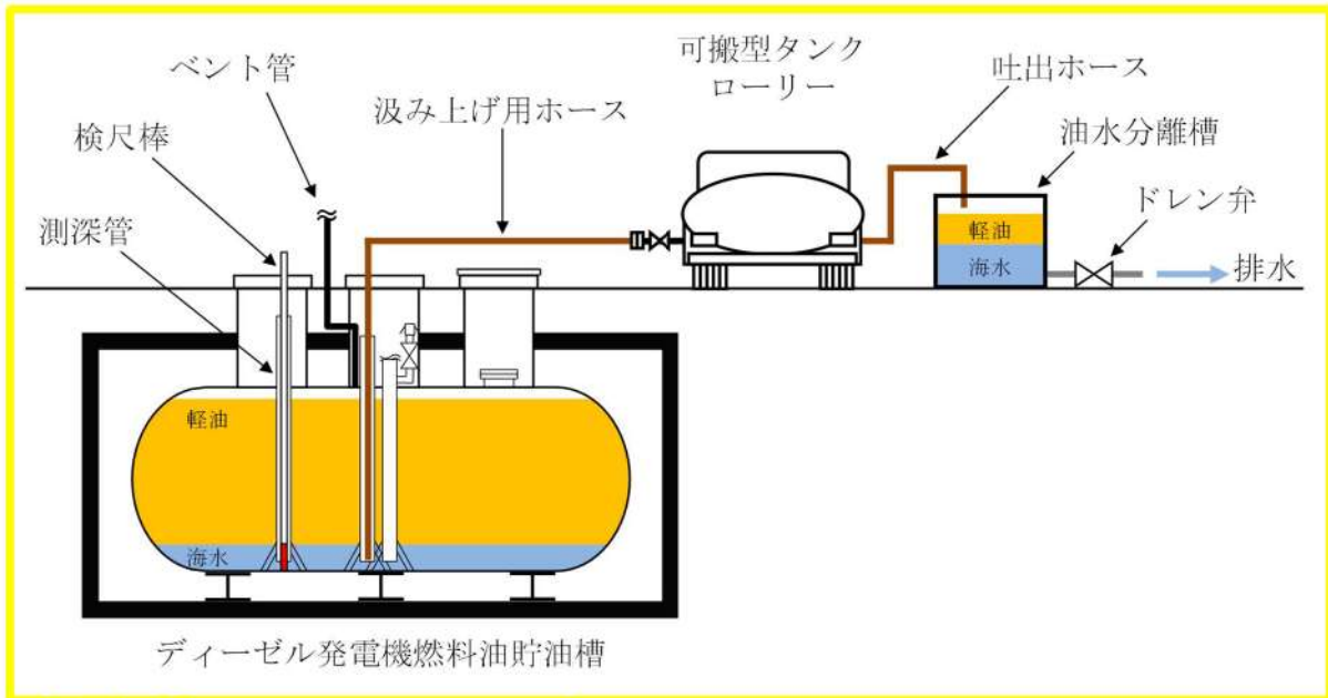
第2図 ディーゼル発電機燃料油貯油槽の軽油と海水の分離方法のイメージ図
